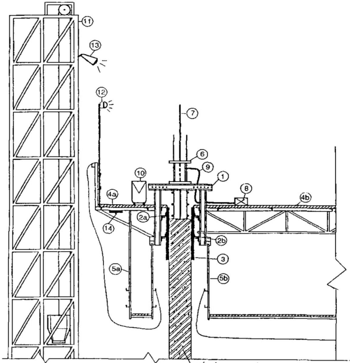
Hình 1. Ví dụ sơ đồ hệ thống cốp pha trượt
