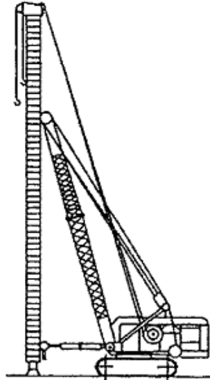
Hình A1.4.2 Máy đóng cọc bánh xích
