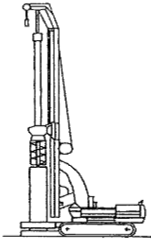
Hình A1.2.4 Máy khoan cọc nhồi chuyên dụng với cơ cấu xoay hạ ống vách.
