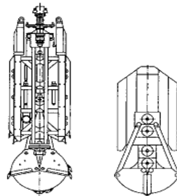
Hình A1.3.2 Gầu ngoạm dùng để thi công tường trong đất, có thể được treo tự do trên cáp hoặc được dẫn theo một dẫn hướng, đóng mở gầu bằng thủy lực hoặc bằng cáp
