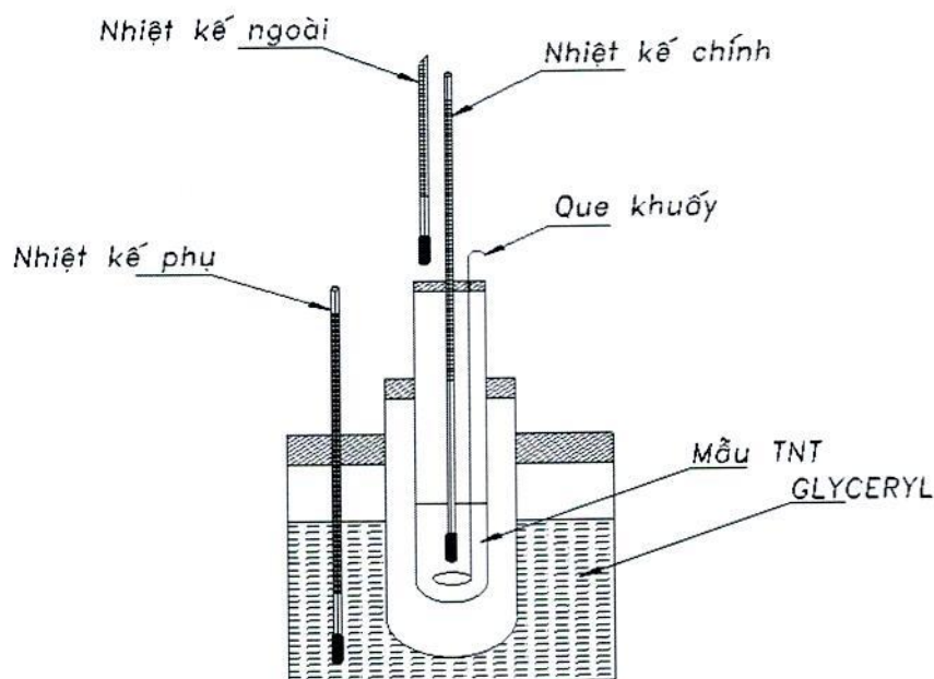
Hình 1. Bộ dụng cụ xác định điểm đông đặc của Trinitrotoluen
