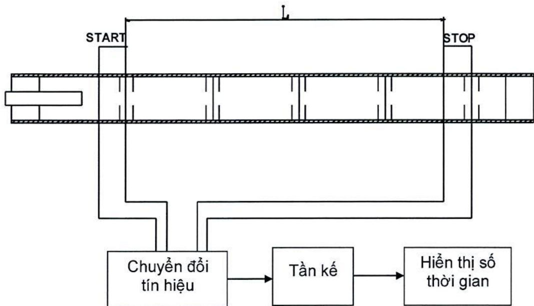
Hình 6. Sơ đồ đấu nối và chuẩn bị đo tốc độ nổ
