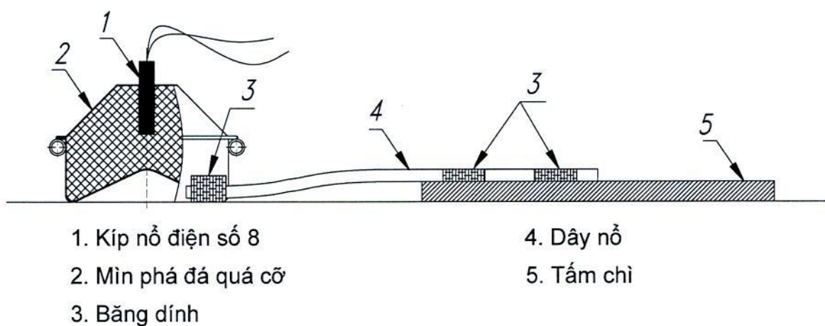
Hình 3 - Sơ đồ xác định độ nhạy kích nổ
