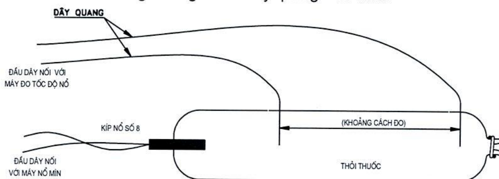
Hình 2 - Sơ đồ chuẩn bị mẫu và cách đấu dây với mẫu thuốc nổ
