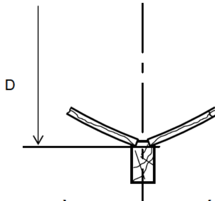
Hình 2 Chiều cao mạn lý thuyết (D) tàu vỏ gỗ
