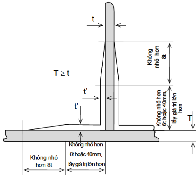
Hình 5.1 Kích thước phần chống của liên kết chữ T
