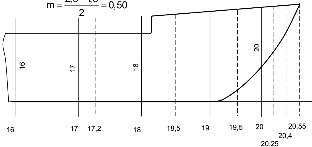
Hình 19 Phân bố sườn phụ và xác định hệ số hiệu chỉnh m trong vùng mũi của tàu
