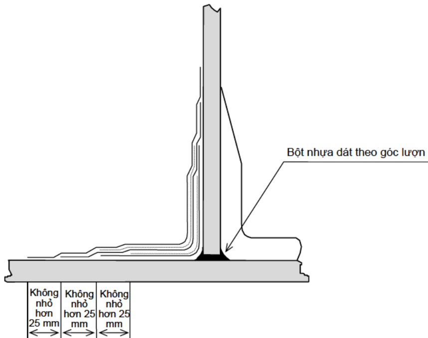
Hình 5.1 Kích thước phần chống của liên kết chữ T
