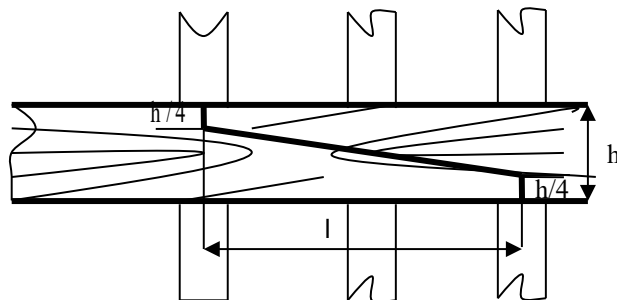
Hình 2/2.4.3-16 - Quy cách mỗi nối gài
