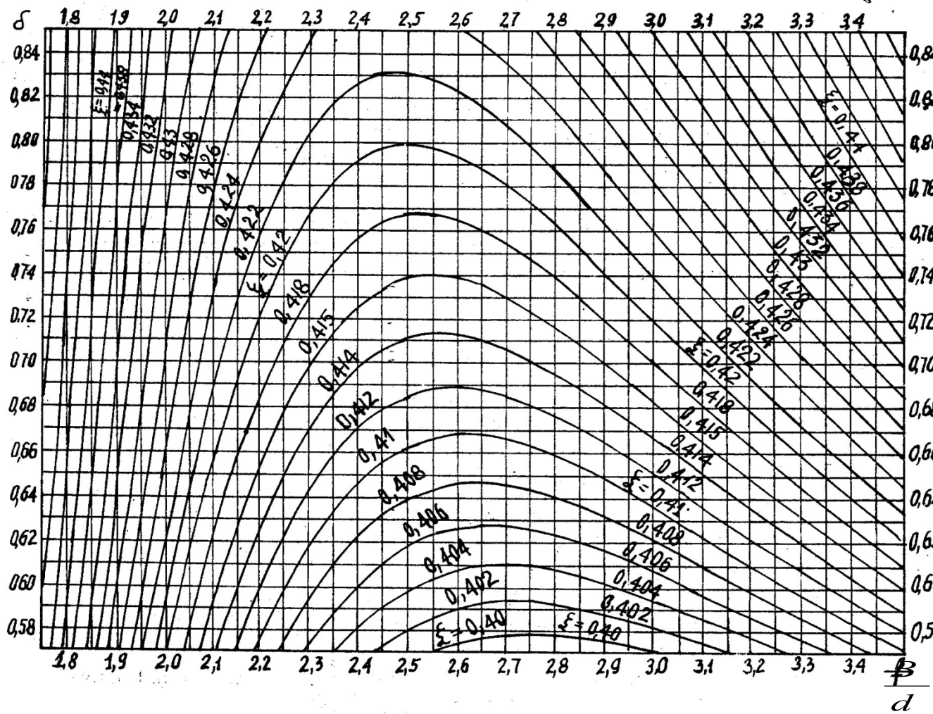
Hình 4/4.4.4 Xác định hệ số \xi
