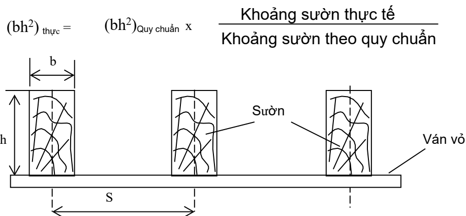
Hình 2/2.4.3-6 - Tiết diện sườn
