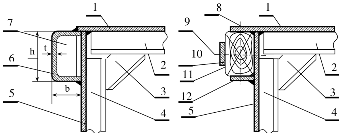
Hình 2/2.3.4-14(1)- Chống va bằng thép
