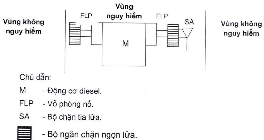
Hình 13. Mô phỏng bộ chặn ngọn lửa
