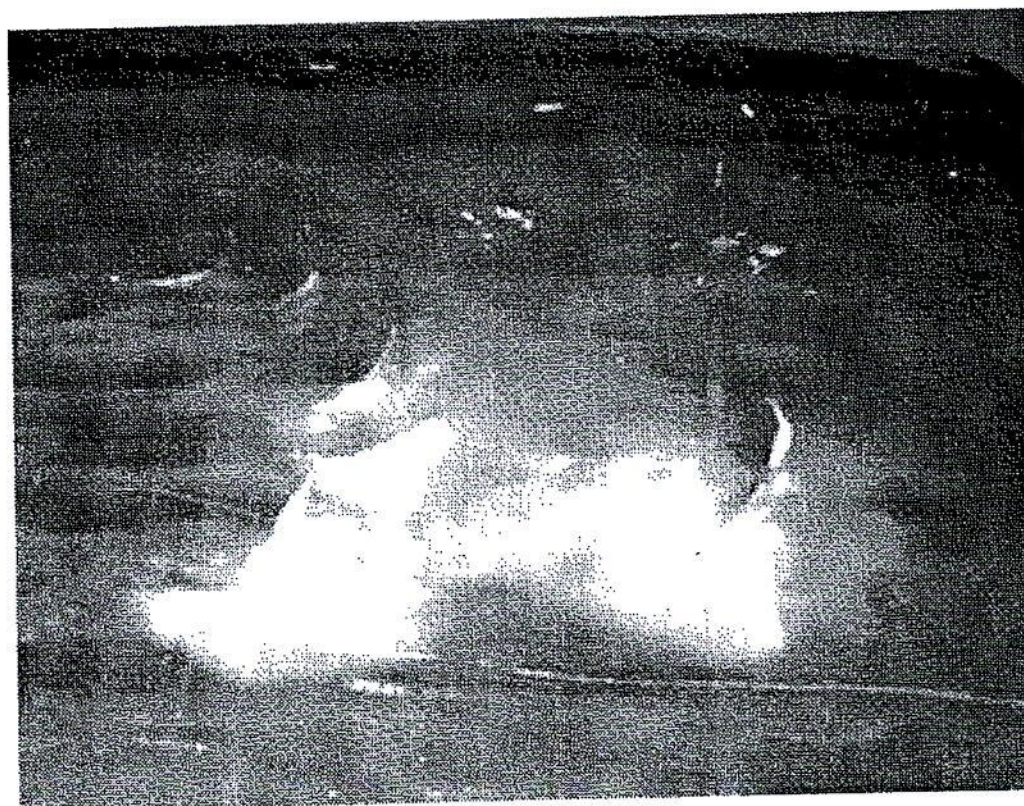
Hình 3. Hư hỏng do va chạm kết hợp giữa tách lớp và khiếm khuyết bề mặt
