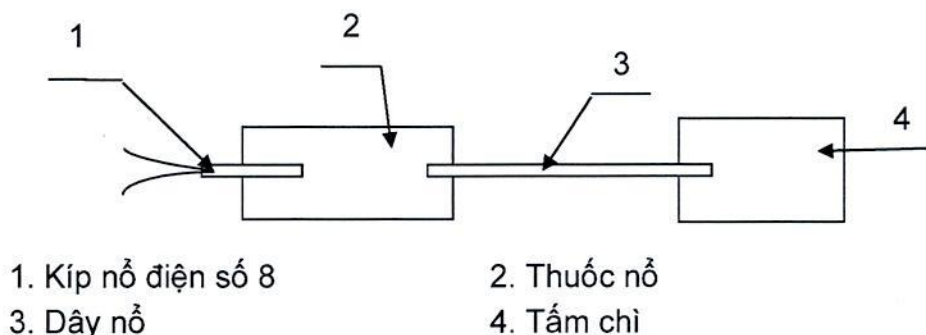
Hình 2 - Sơ đồ xác định độ nhạy kích nổ
