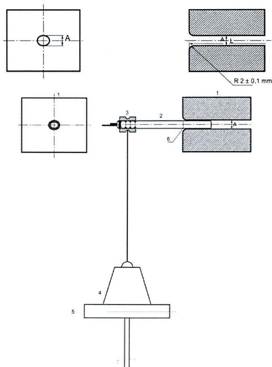
Hình 1. Thiết bị khả năng chống uốn của kíp
