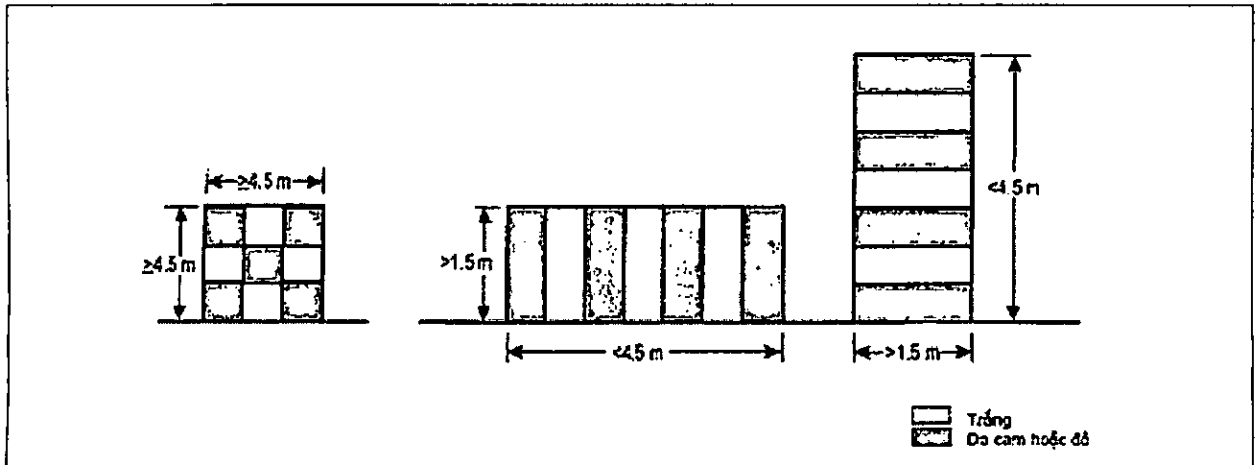
Hình 1-PLIV. Mẫu sơn, kẻ cơ bản
