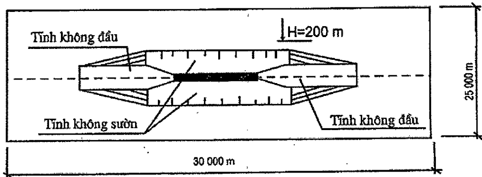
Hình 7-PLI: Vùng phụ cận đường sân bay
