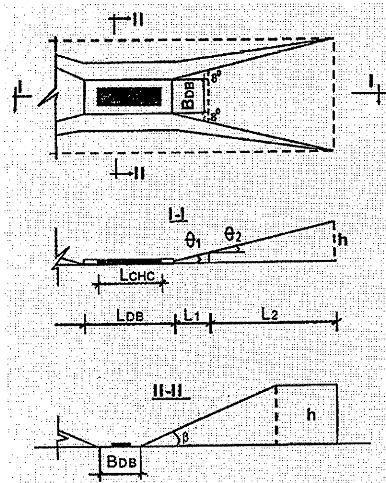
Hình 5-PLI. Sơ đồ kích thước dải bay và giới hạn độ cao chương ngại vật đối với bãi cát, hạ cánh
