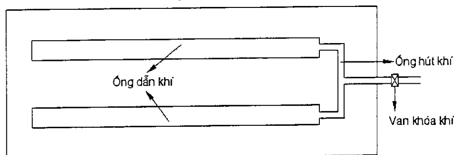
Hình 1: Mô hình kiểu một cửa hút khí song song
