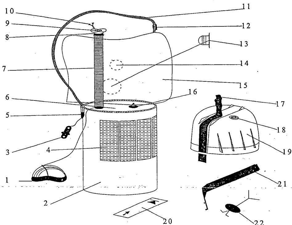
Hình 2 - Cấu tạo mẫu của bình tự cứu cá nhân dạng cách ly Chỉ dẫn cấu tạo mẫu của bình tự cứu cá nhân dạng cách ly
