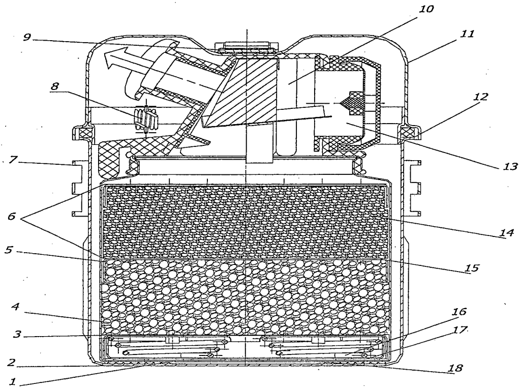
Hình 1 - Cấu tạo mẫu của bình tự cứu cá nhân dạng hấp thụ Chỉ dẫn cấu tạo mẫu của bình tự cứu cá nhân dạng hấp thụ
