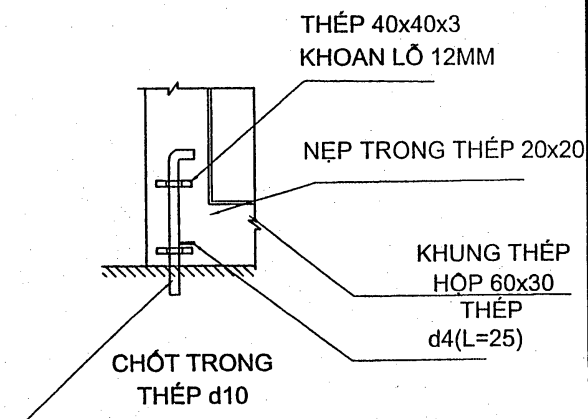
CHI TIẾT CHỐT ĐỨNG
