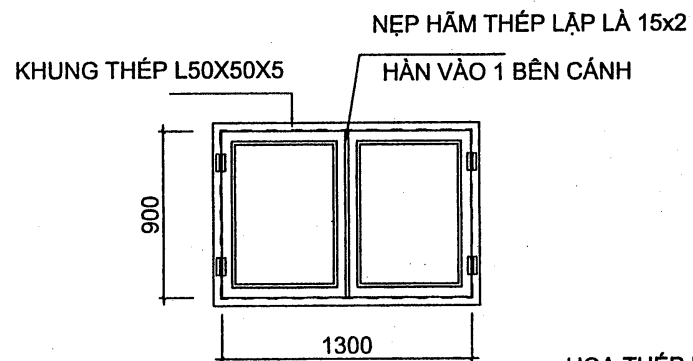
CỬA SỔ (LỚP CỬA BÊN NGOÀI) NHÀ KHO
