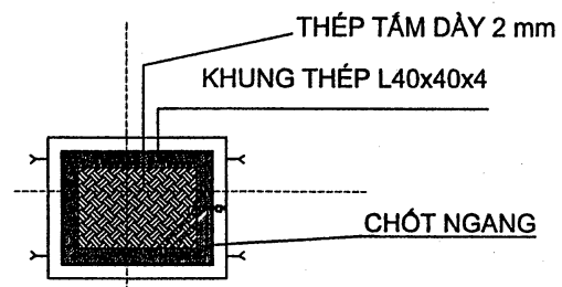
MẶT CHIẾU ĐỨNG CÁNH CỬA THÔNG GIÓ NỀN
