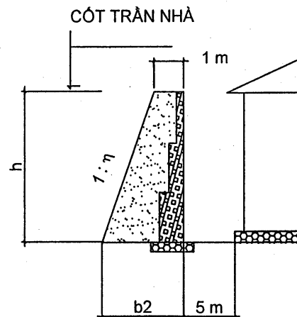
2. Ụ ĐẮP ĐẤT CÓ KÈ MỘT BÊN (BẰNG BÊ TÔNG CỐT THÉP)
