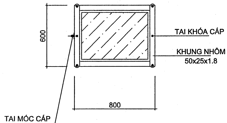
CT SONG SẮT CỬA THÔNG GIÓ TRẦN NHÀ KHO
