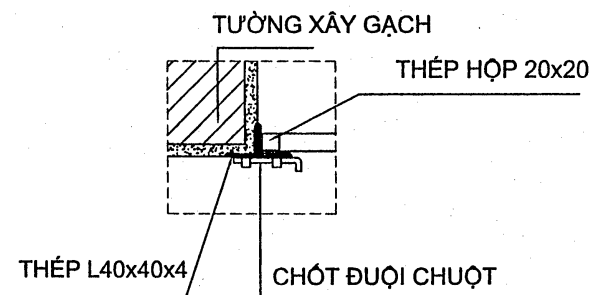
CHI TIẾT CHÓT NGANG
