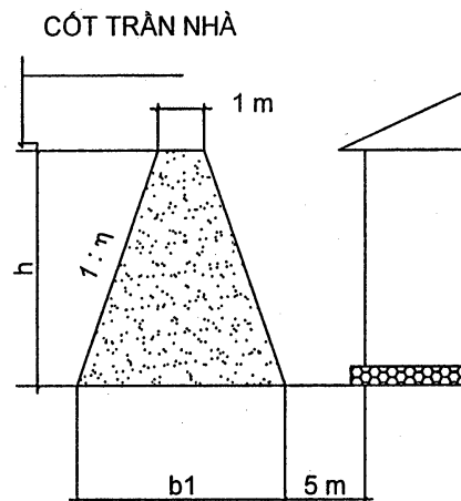
1. Ụ ĐẮP ĐẤT
