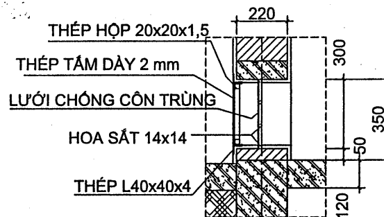
MẶT CẮT ĐỨNG CỬA THÔNG GIÓ NỀN
