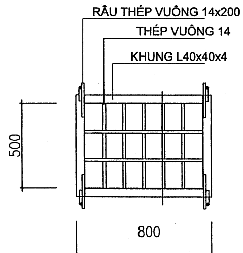
CT SONG SẮT CỬA THÔNG GIÓ TRẦN NHÀ KHO
