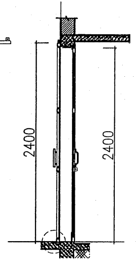
MẶT CẮT 1 - 1
