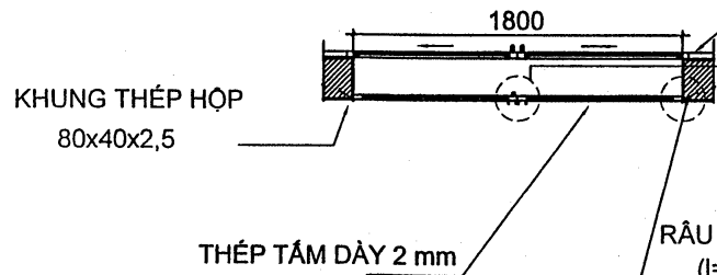
MẶT CẮT 1 - 1
