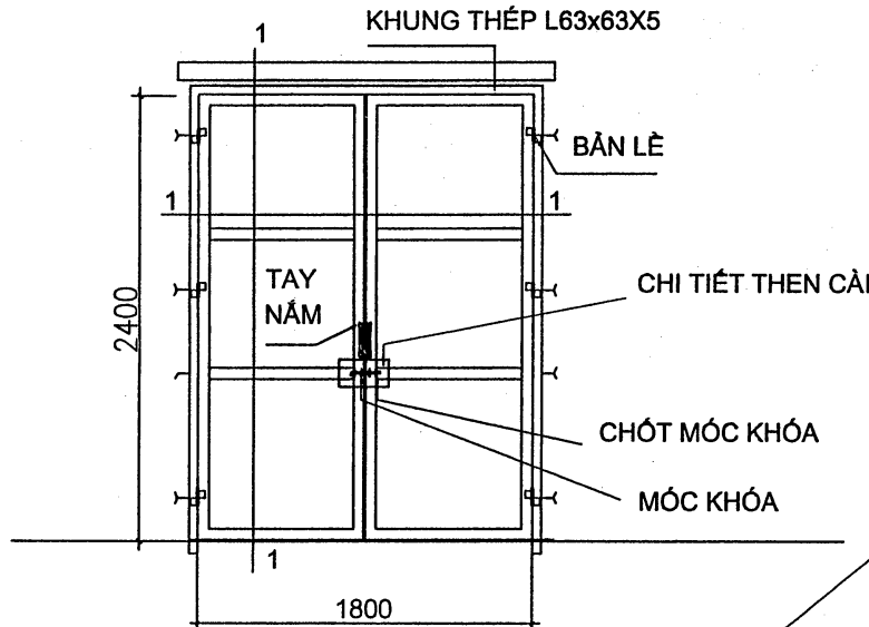
CỬA RA VÀO (LỚP CỬA BÊN NGOÀI)
