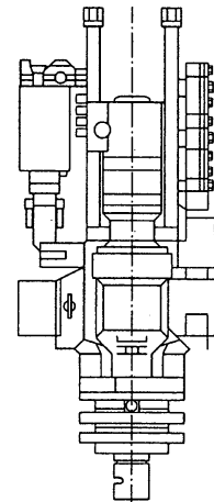
Hình A1.2.9 Búa khoan kiểu xoay va đập
