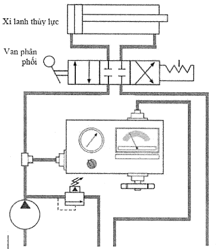
Hình B4 Sơ đồ lắp bộ thiết bị kiểm tra hoạt động và độ kín trong của xi lanh thủy lực và van phân phối
