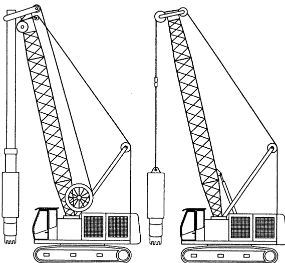
Hình A1.3.1 Máy thi công tường trong đất: Thủy lực và rơi tự do
