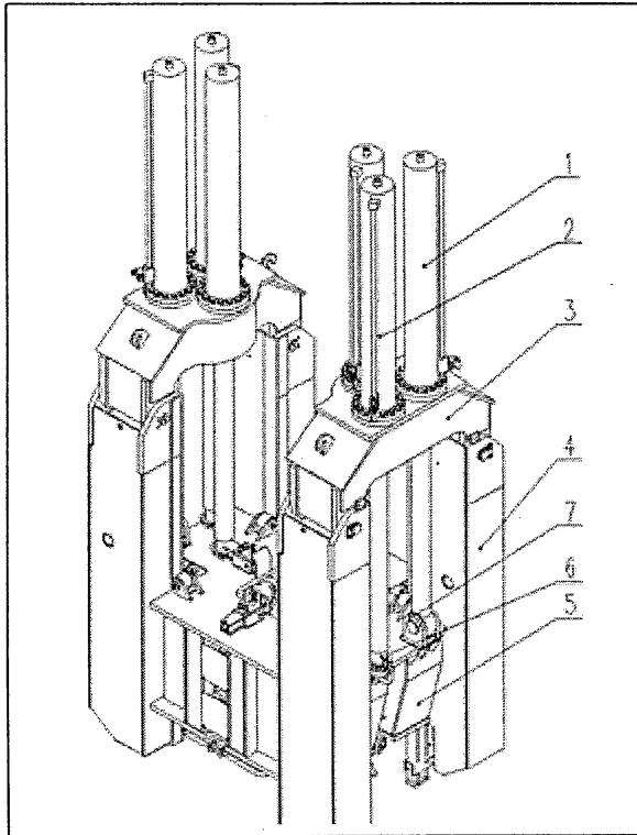
Hình A2.2.2 Cấu tạo của cơ cấu ép cọc: 1, 2 – Các xi lanh thủy lực ép cọc (chính và phụ); 3 – Dầm ngang đỡ các xi lanh thủy lực ép cọc; 4 – Trụ đứng dẫn hướng ép cọc; 5 - Hộp kẹp cọc; 6 - Ấc và chốt ghép cần của xi lanh thủy lực ép cọc với hộp kẹp cọc; 7 – Bát cầu trên hộp kẹp cọc 5 có nhiệm vụ tiếp nhận đầu dạng cầu tròn của các xi lanh thủy lực ép cọc phụ
