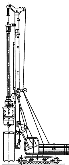
Hình A1.2.2 Máy khoan cọc nhồi chuyên dụng với cần khoan Kelly và gầu khoan
