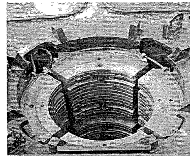
Hình A2.2.4 Hộp kẹp cọc với chấu ôm cọc tròn dùng để ép cọc tròn
