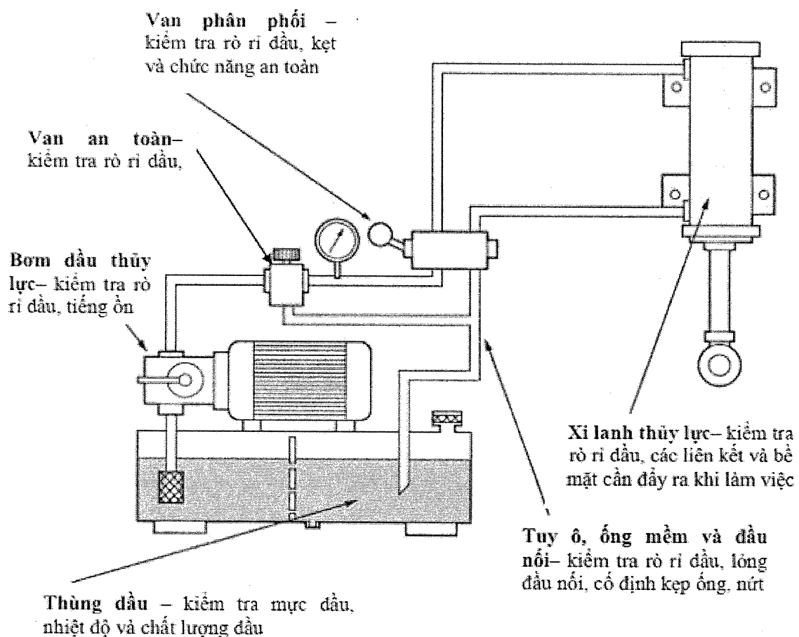
Hình B1 Sơ đồ hệ thống dẫn động thủy lực máy ép cọc với các phần tử thủy lực được coi là quan trọng và chỉ dẫn kiểm tra rò rỉ bên ngoài bằng trực quan
