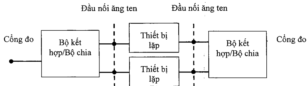
Hình A.1 - Ví dụ về cấu hình thiết bị thiết bị lắp.
