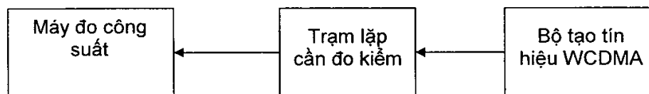
Hình D.1 - Sơ đồ đo công suất ra cực đại
