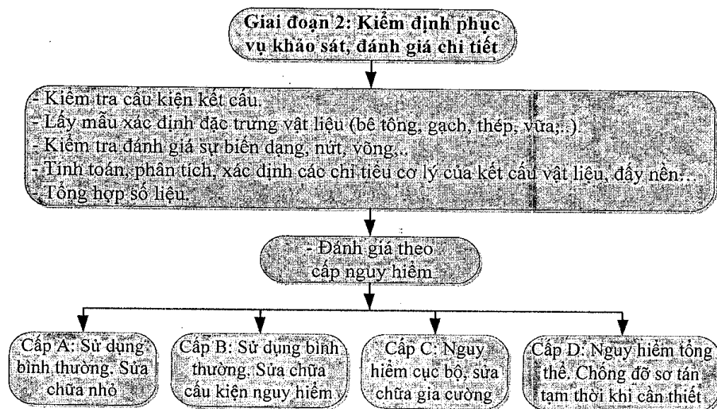
Sơ đồ 2. Trình tự và nội dung chủ yếu của Giai đoạn 2 (Kiểm định phục vụ khảo sát, đánh giá chi tiết)
