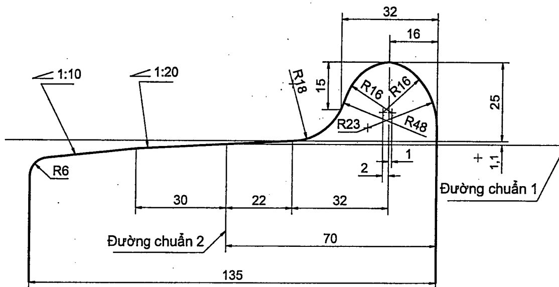
Hình A.3. Biên dạng mặt lăn côn khổ đường 1.435 mm
