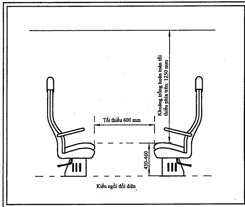
Hình 6: Khoảng không gian của ghế loại đối diện
