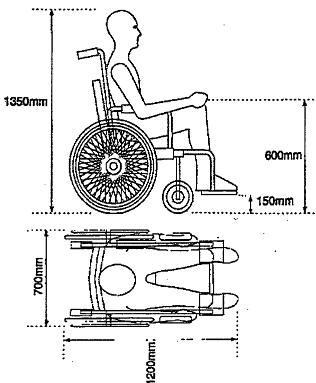
Hình 1: Xe lăn chuẩn
