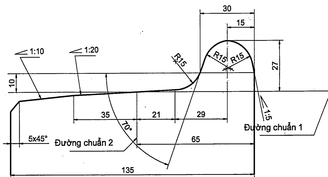
Hình A.2. Biên dạng mặt lăn côn khổ đường 1.000 mm
