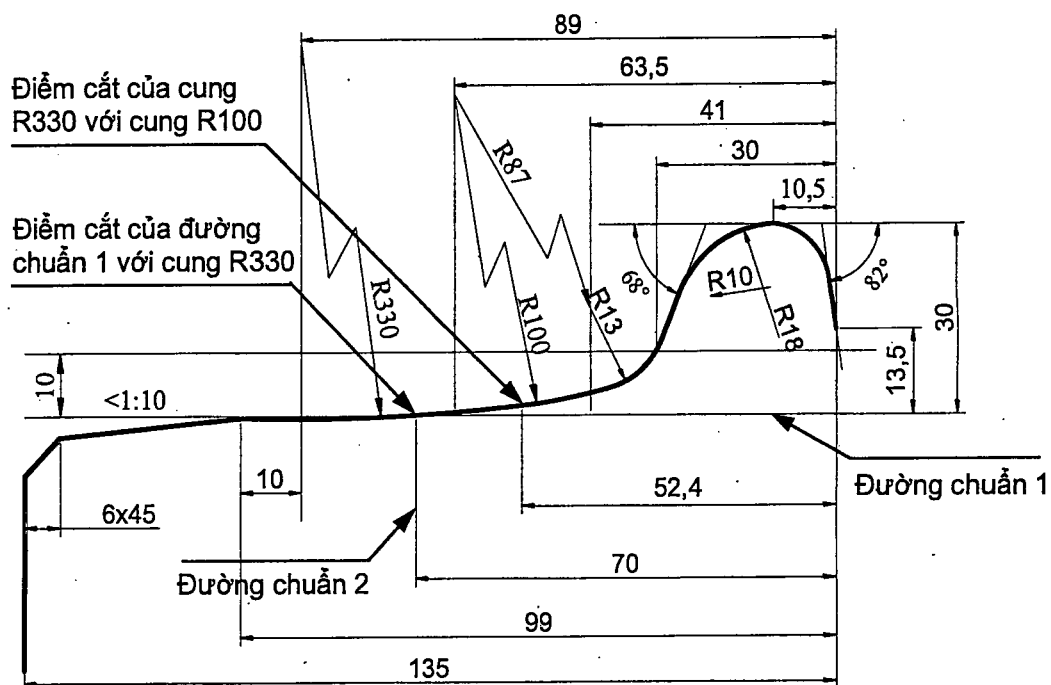
Hình A.1 – Biên dạng mặt lăn lổm khổ đường 1000 mm
