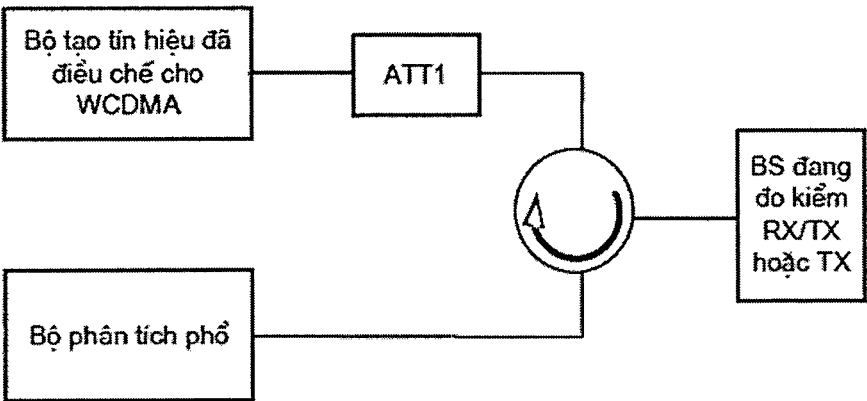
Hình D.4 - Sơ đồ đo xuyên điều chế phát của trạm gốc
