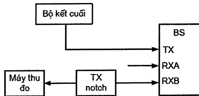
Hình D.6 - Sơ đồ đo phát xạ giả của máy thu
