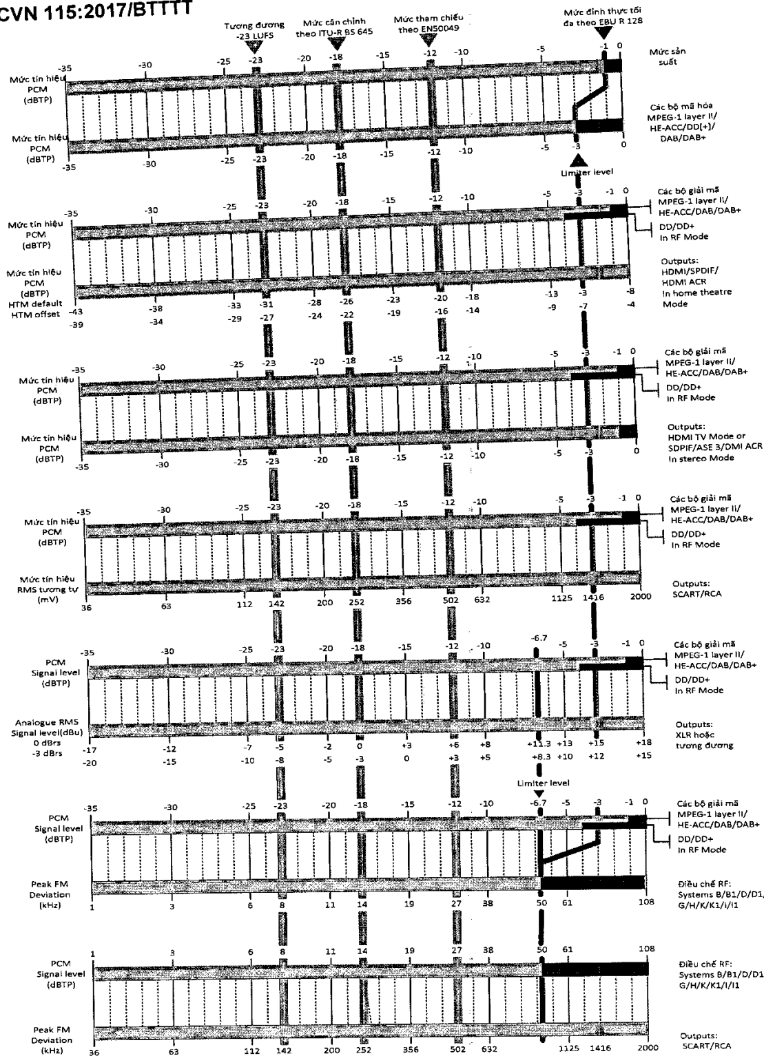
Hình B.8 - Cân chỉnh mức trong các hệ thống B, B1, D, D1, G, H, K, K1, I và I1
