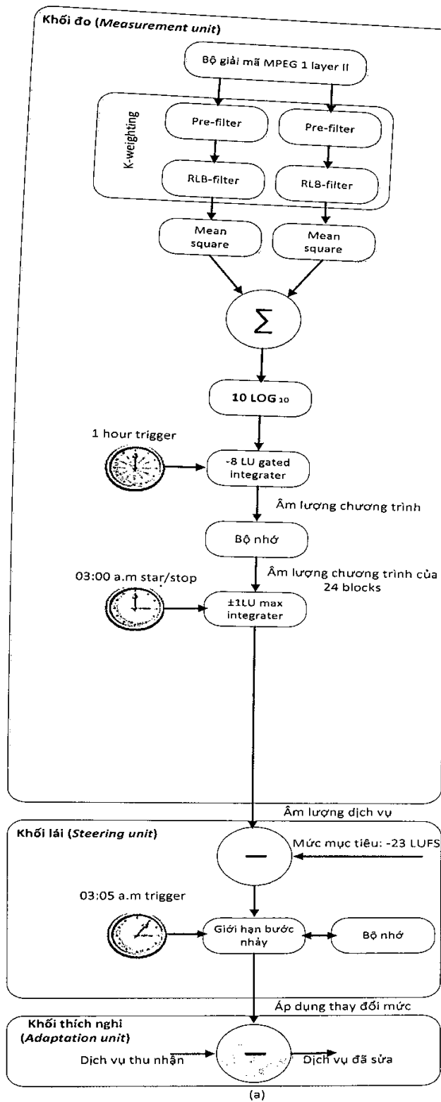
Hình B.2 biểu diễn sơ đồ đo âm lượng và cách thức chuẩn hóa cho các dịch vụ với mã hóa khác nhau. QCVN 115:2017/BTTTT
