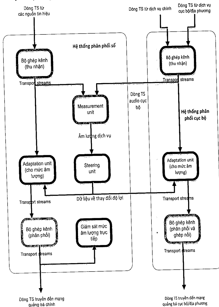
Hình B.6 - Sơ đồ khối của head-end số tích hợp chuẩn hóa âm lượng và một head-end cục bộ thực hiện thay một dịch vụ trong dòng truyền chính bởi dịch vụ khu vực
