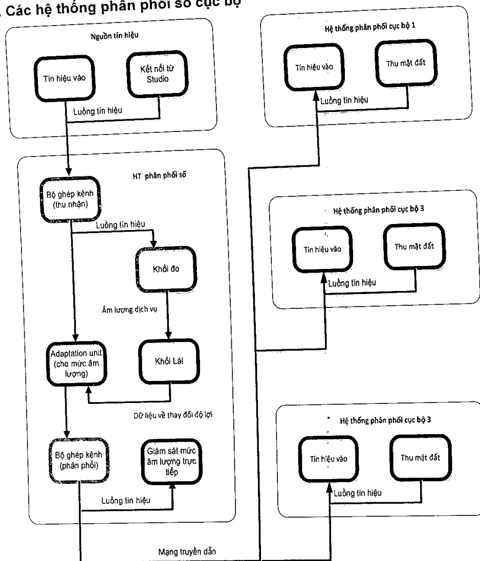
Hình B.3 - Mô hình phân phối âm thanh chuẩn hóa từ hệ thống phân phối trung tâm đến các hệ thống phân phối cục bộ
