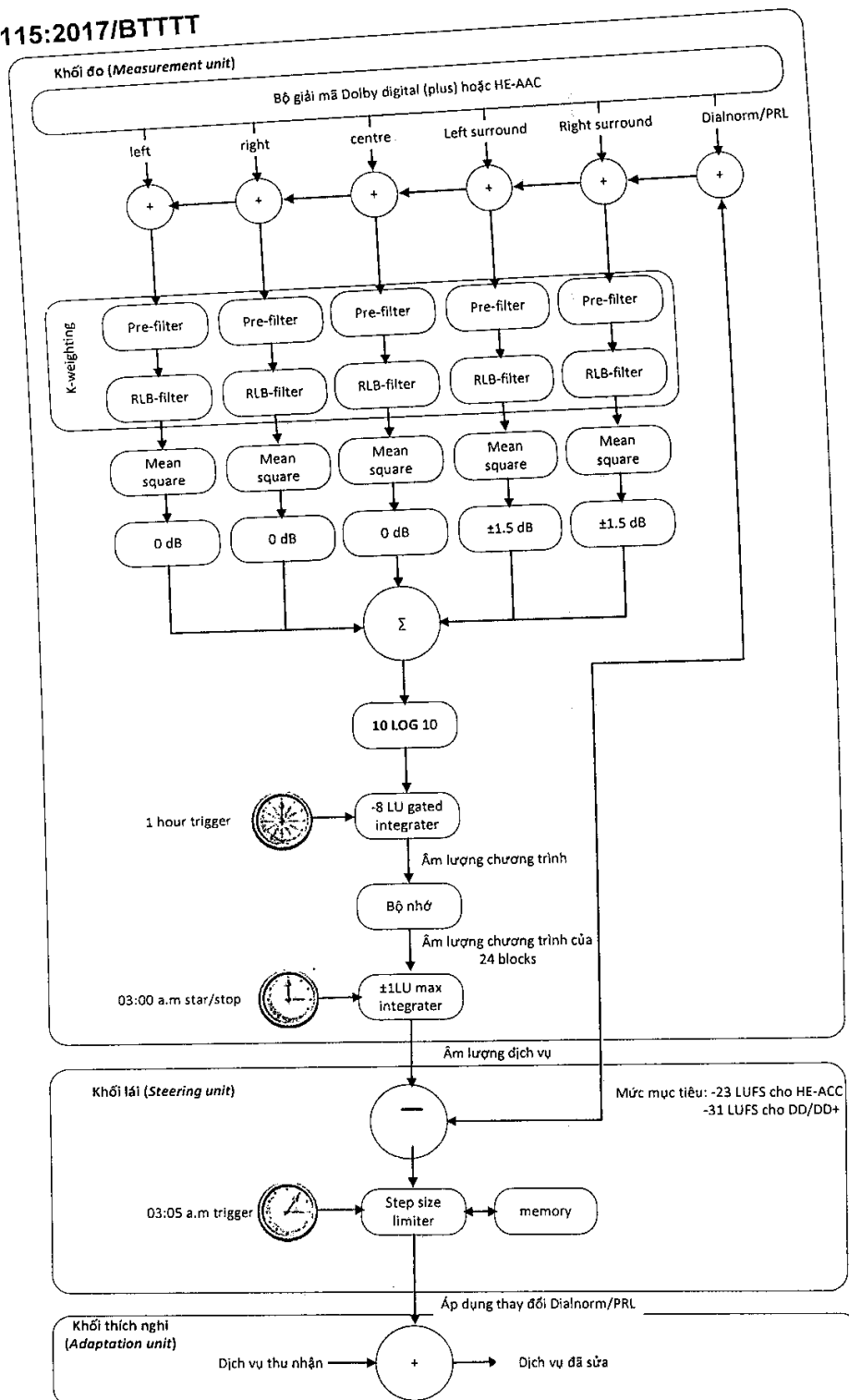
Hình B.2- Sơ đồ khối quá trình đo các dịch vụ ứng với các mã hóa sử dụng (a) MPEG-1 Layer II; (b) DD/DD+ và/hoặc HE-AAC
