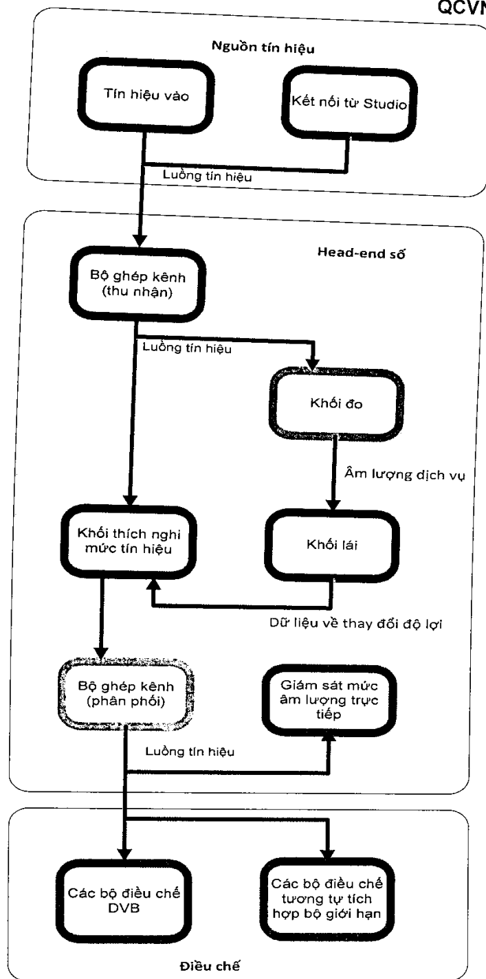
Hình B.1- Mô hình hệ thống phân phối tích hợp chuẩn hóa âm lượng
