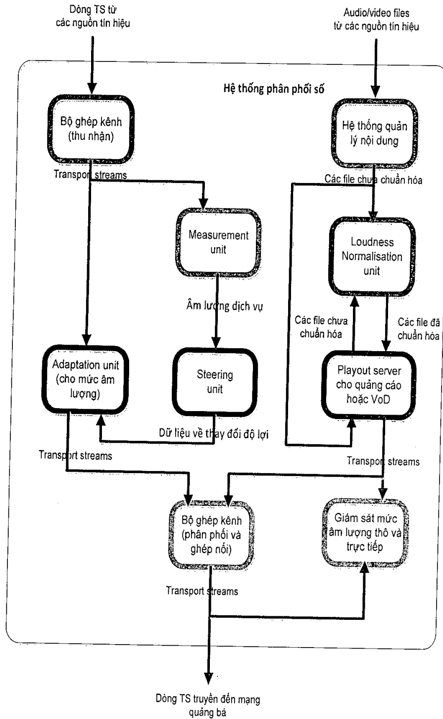
Hình B.5 - Sơ đồ khối một hệ thống phân phối số tích hợp chuẩn hóa âm lượng cho VoD và chèn quảng cáo
