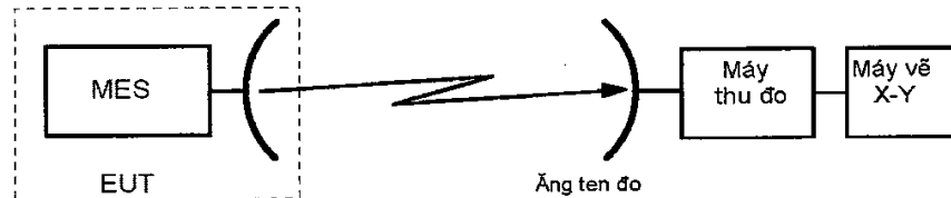
Hình 15 - Sơ đồ đo giản đồ bức xạ phát của ăng ten
