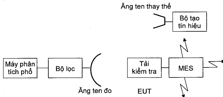
Hình 5 - Sơ đồ đo phát xạ không mong muốn của EUT khi không có ăng ten
