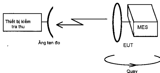
Hình 1- Sơ đồ đo phát xạ không mong muốn, trực đầu tiên
