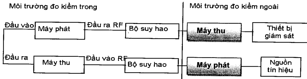
Hình 5 - Cấu hình đo kiểm cho máy thu phát
