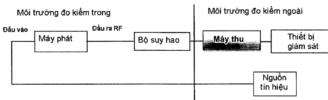
Hình 3 - Cấu hình đo kiểm cho máy phát
