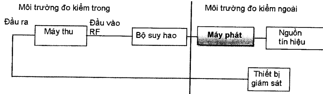
Hình 4 - Cấu hình đo kiểm cho máy thu
