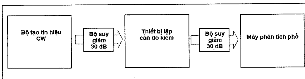
Hình C. 2 – Sơ đồ đo tăng ích ngoài băng
