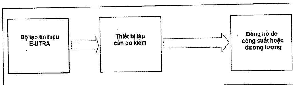
Hình C. 1 – Sơ đồ đo công suất cực đại
