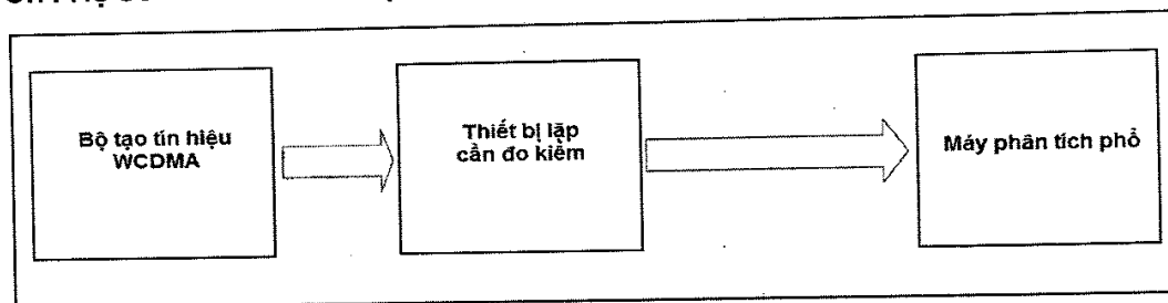
Hình C. 7 – Sơ đồ đo hệ số nén kênh lân cận
