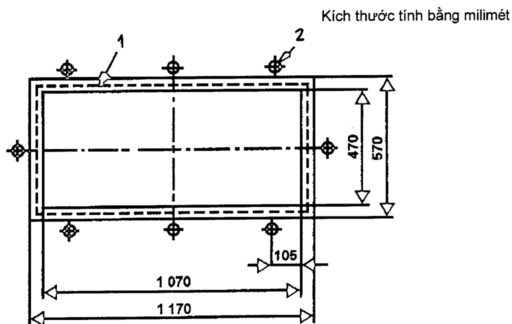
Hình 3 - Giá đỡ thử bằng chùy thử
