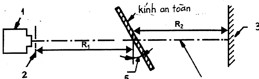
Hình 11 - Sơ đồ bố trí thử độ méo quang học
