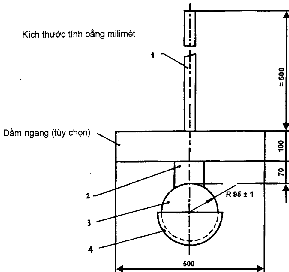
Hình 2. Chùy thử
