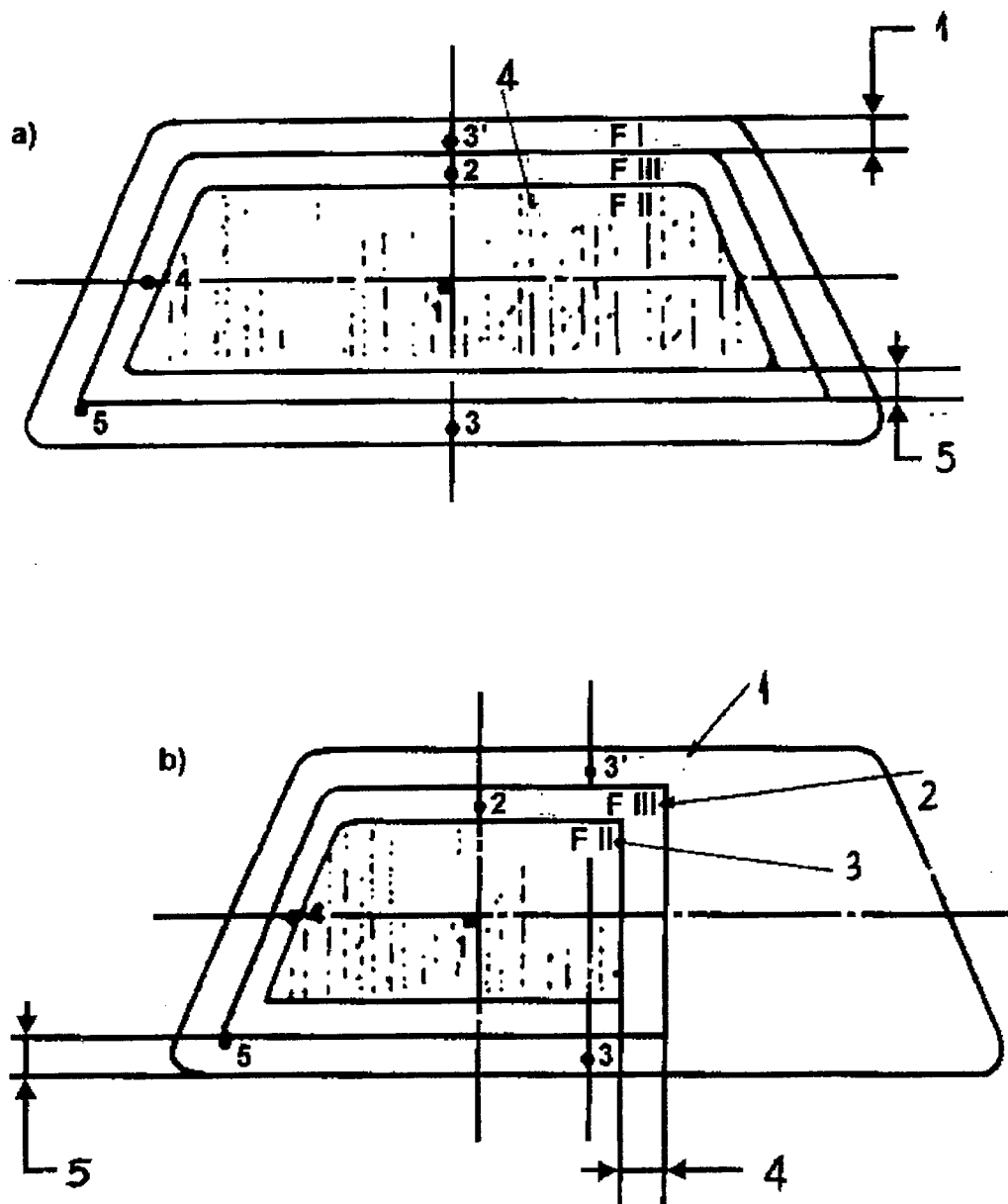
Hình 2 - Các điểm và đập quy định cho kính chắn gió
