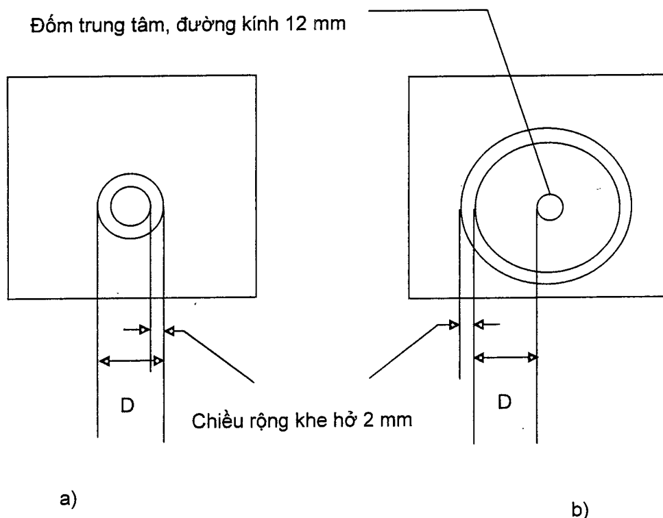
Hình 13 - Các kích thước của bia
