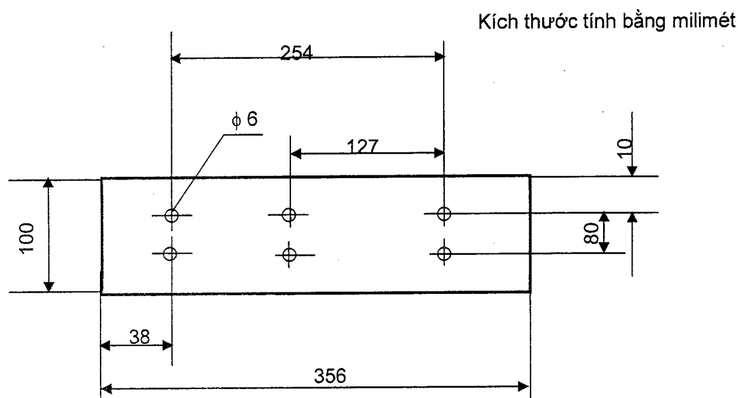
Hình 22 - Mẫu thử
