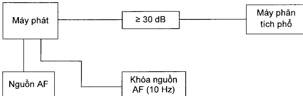
Hình 4 – Sơ đồ đo đặc điểm tần số quá độ của máy phát
