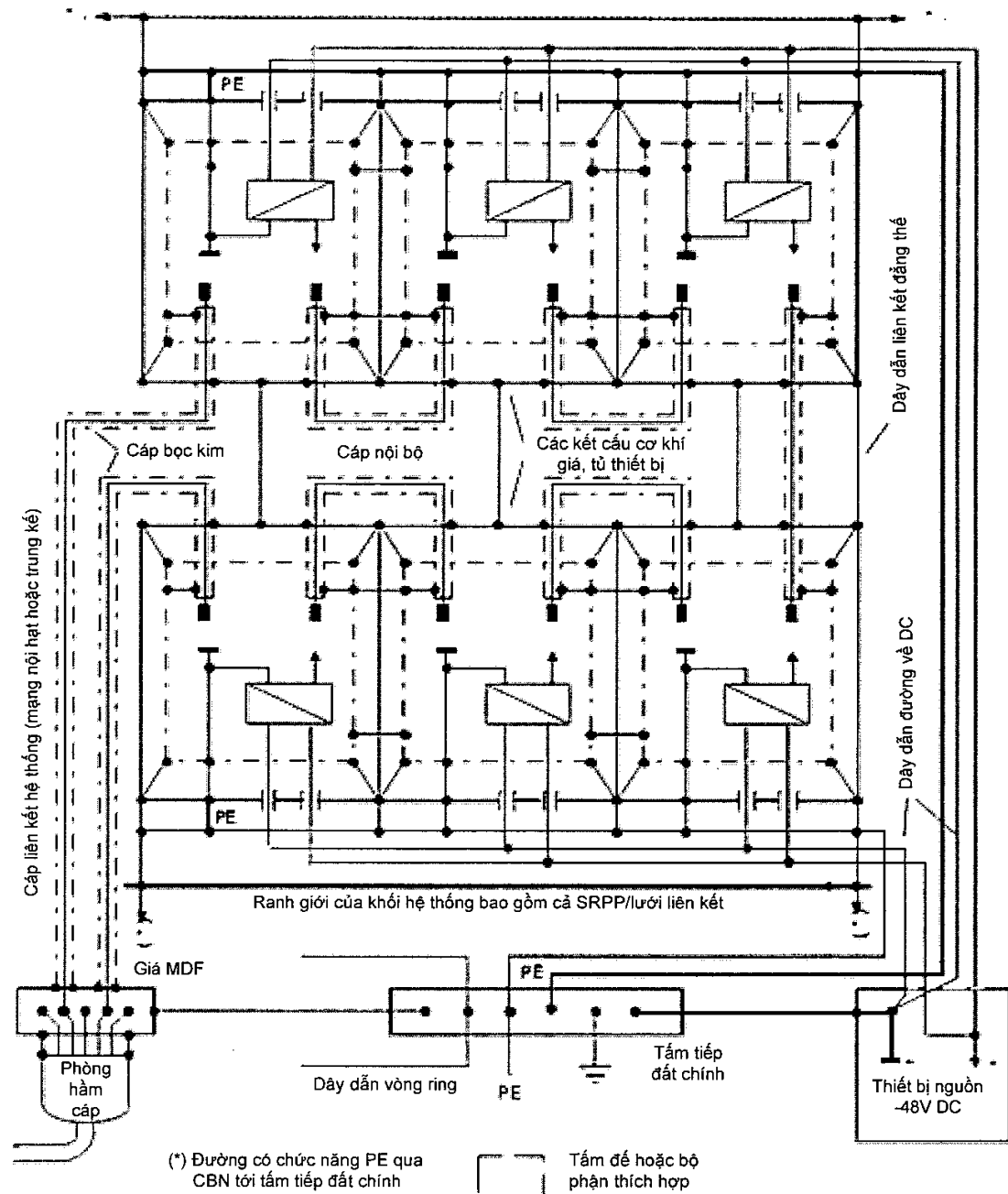
Hình 4 - CBN/ MESH-BN với đường về DC cách ly, nối với CBN tại một điểm
