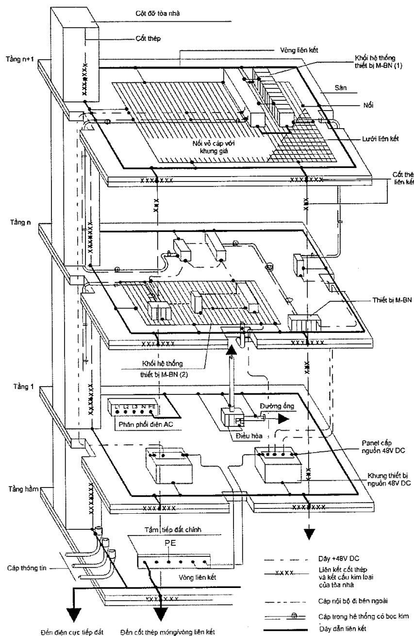
Hình 2 - Mạng MESH- BN kết nối với CBN
