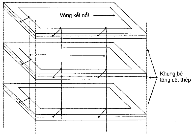
Hình 1 - Mạng CBN
