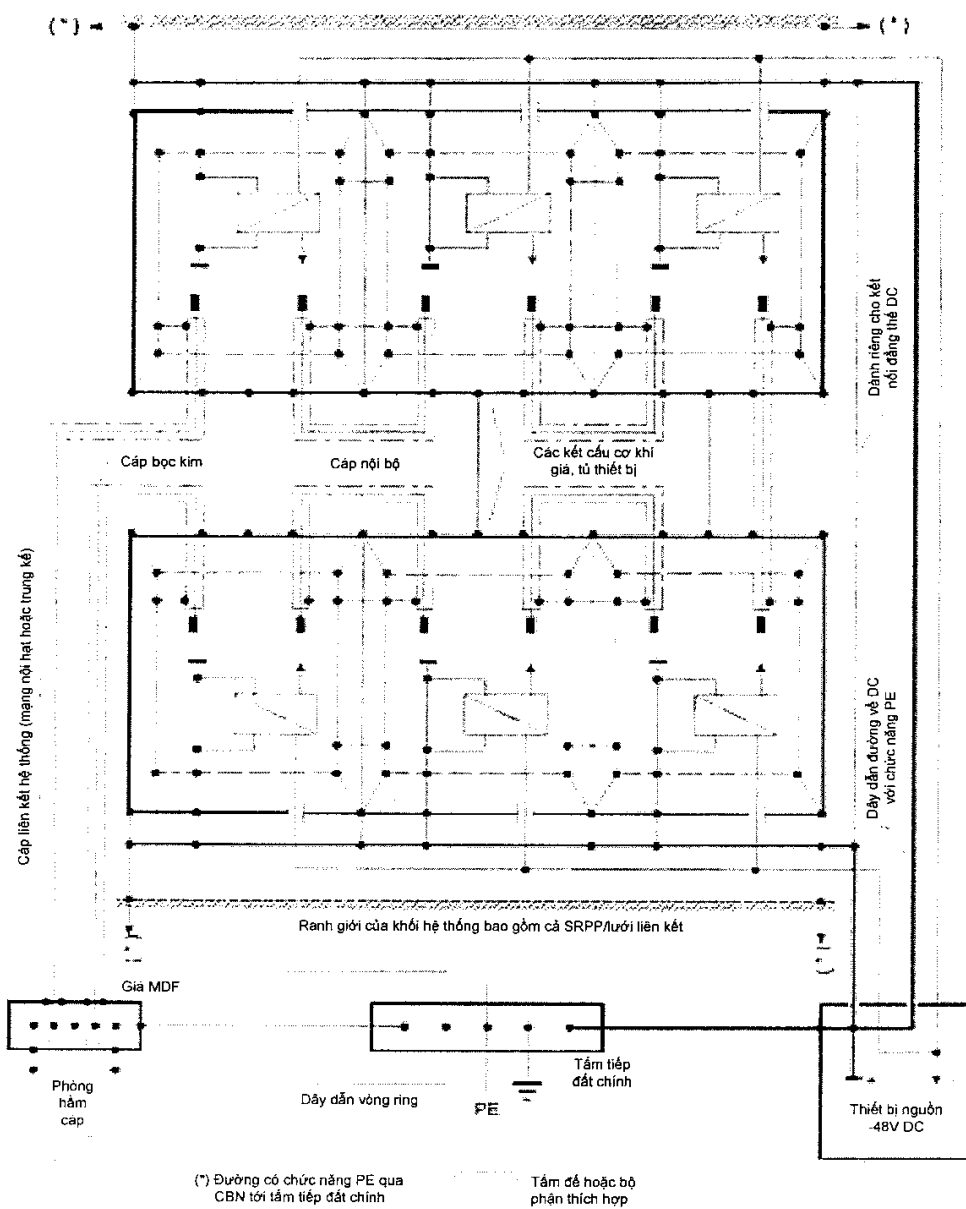
Hình 3 - CBN/MESH-BN với đường về DC chung nối với CBN tại nhiều điểm
