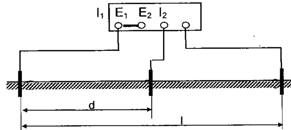
Hình A.1 - Sơ đồ đo điện trở tiếp đất
