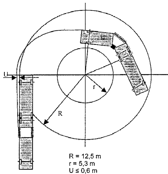
Hình 6b - Khả năng quay vòng xe nối toa
