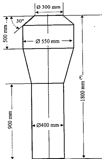
Hình 3 - Đường kiểm tra lối đi dọc
