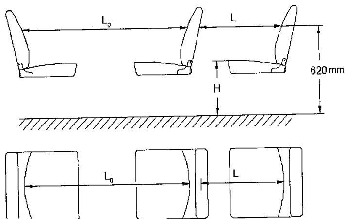
Hình 2 - Kích thước giữa các ghế
