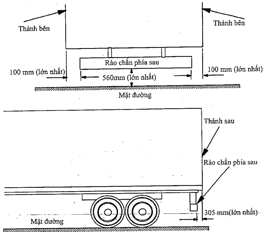
Hình 2: Minh họa yêu cầu đối với rào chắn phía sau
