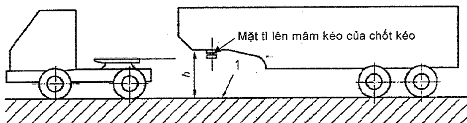
Hình 3: Chiều cao mặt tì lên mâm kéo của chốt kéo
