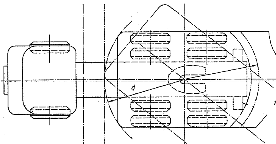
Hình 4: Bán kính khoảng sáng quay đầu phía trước của sơ mi rơ moóc
