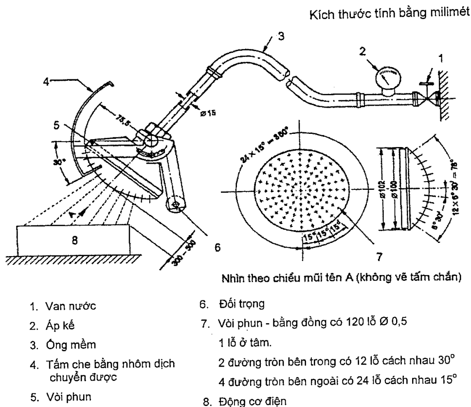
Hình 2. Thiết bị cầm tay để thử nghiệm về bảo vệ chống tia nước
