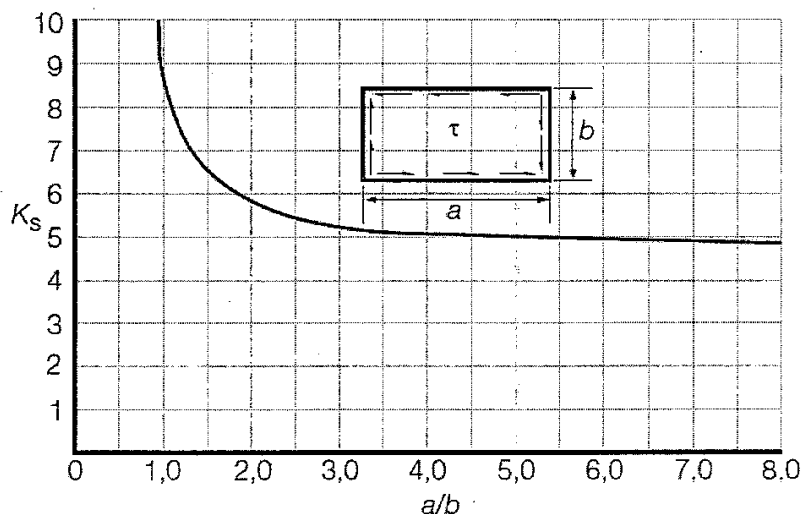
Hình 3.1.2-2 Hệ số K_s
