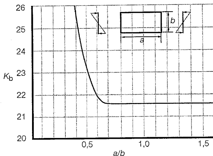
Hình 3.1.2-3 Hệ số K_b
