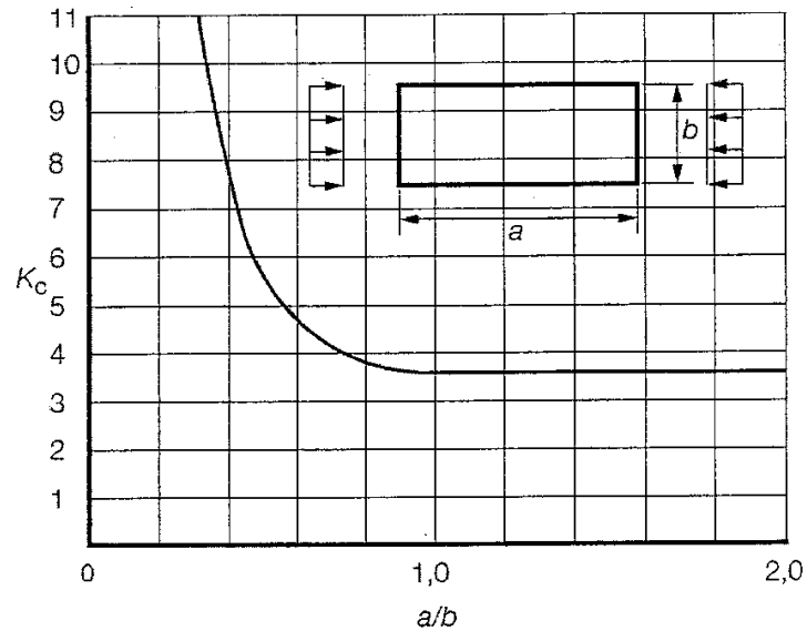
Hình 3.1.2-1 Hệ số K_c
