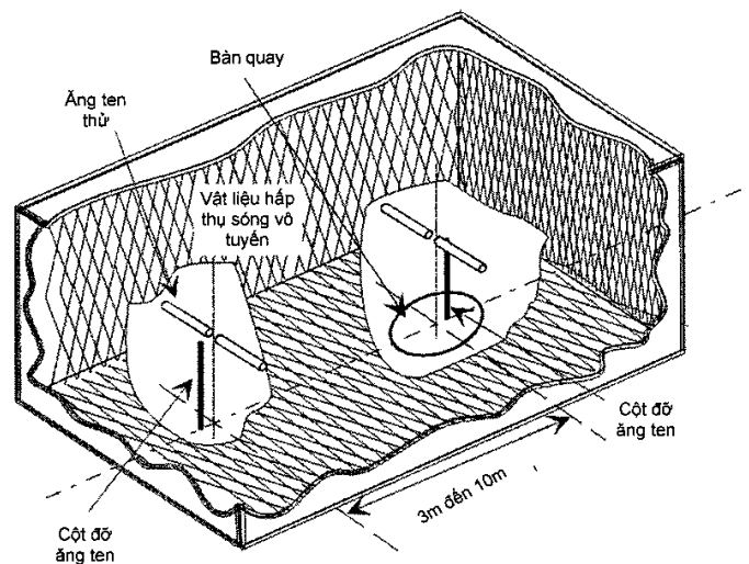
Hình A.1- Buồng đo hấp thụ
