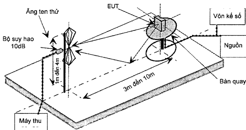
Hình A.4 - Bố trí phép đo tại vị trí đo có mặt nền dẫn (Thiết lập OATS đối với đo kiểm phát xạ giả)
