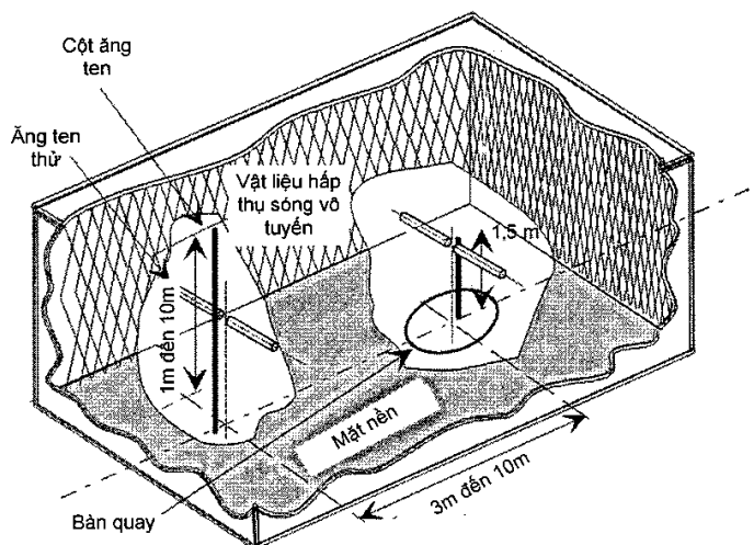
Hình A.2- Buồng đo hấp thụ có mặt nền dẫn
