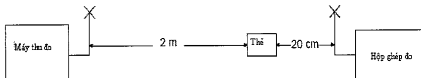
Hình 5 - Sơ đồ đo phát xạ thẻ
