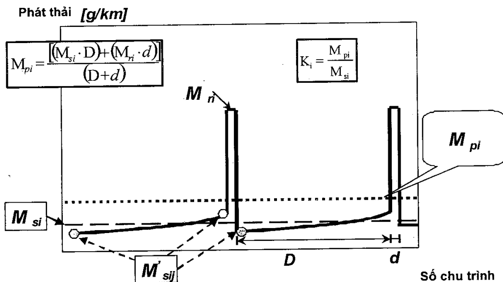
Hình 1. Các thông số cần đo khi thử nghiệm, trong khi và giữa các chu trình xảy ra quá trình tái sinh.
