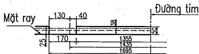
Chi tiết giới hạn tiếp giáp ray
