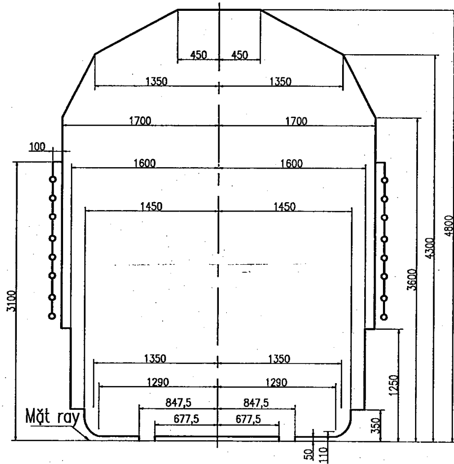
Chi tiết giới hạn tiếp giáp ray
