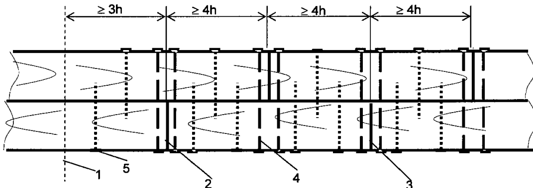
Hình 9 - Mối nối dùng đoạn gỗ táp
