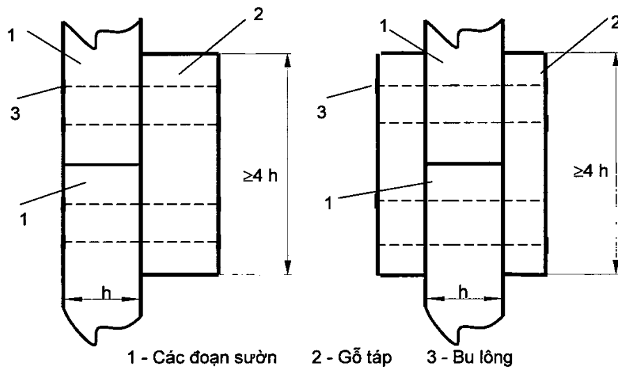
Hình 9 - Mối nối dùng đoạn gỗ táp
