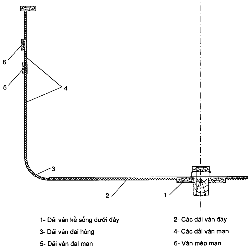
Hình 6 - Các thành phần ván vò
