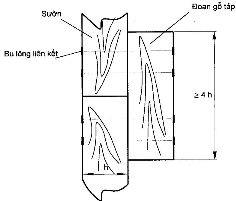
Hình 4 - Mối nối táp sườn đơn
