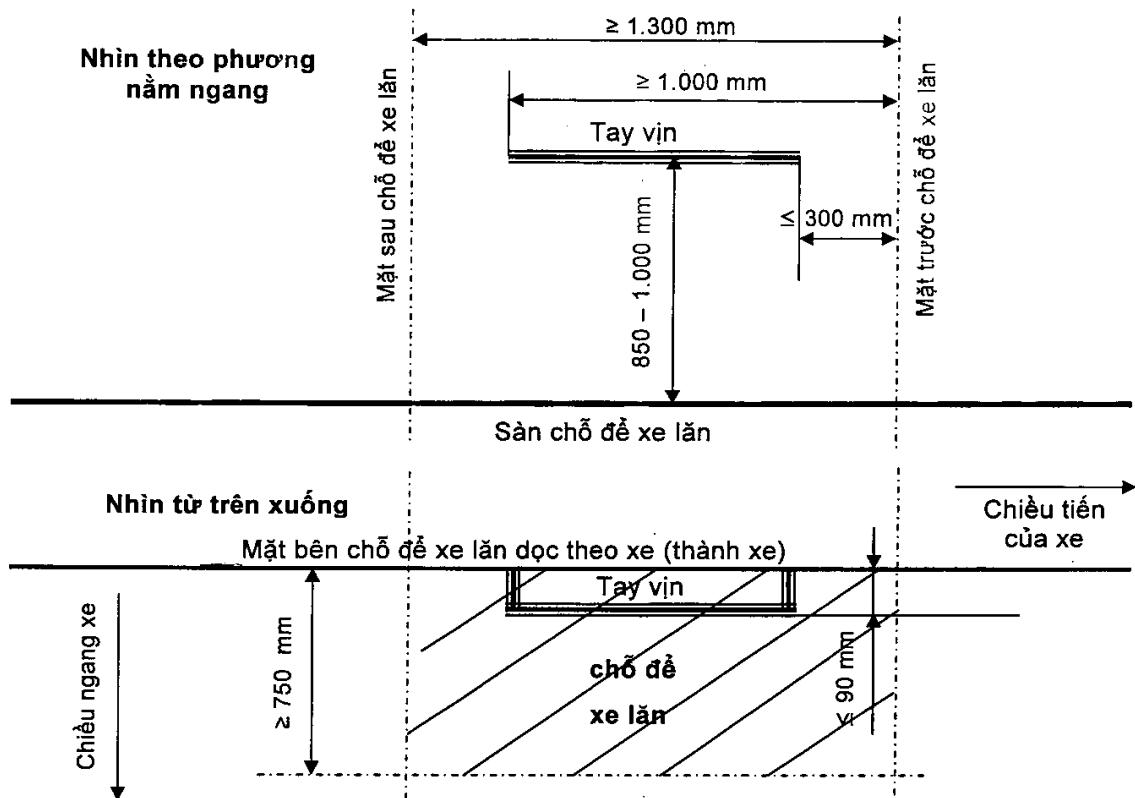
Hình 3. Bố trí tay vịn
