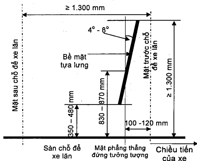
Hình 2. Bố trí tựa lưng
