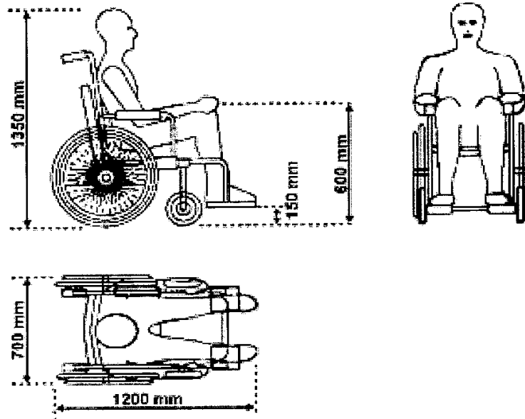
Hình 1. Xe lăn chuẩn
