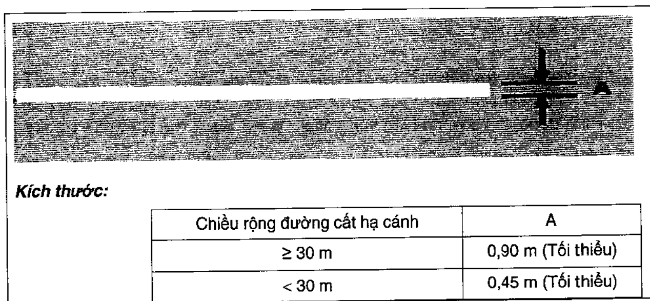
Hình 8 - Sơn tín hiệu cạnh đường cát hạ cánh
