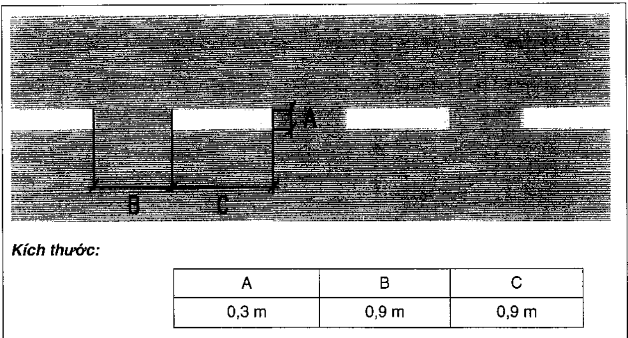
Hình 17 - Sơn tín hiệu vị trí chờ lặn trung gian
