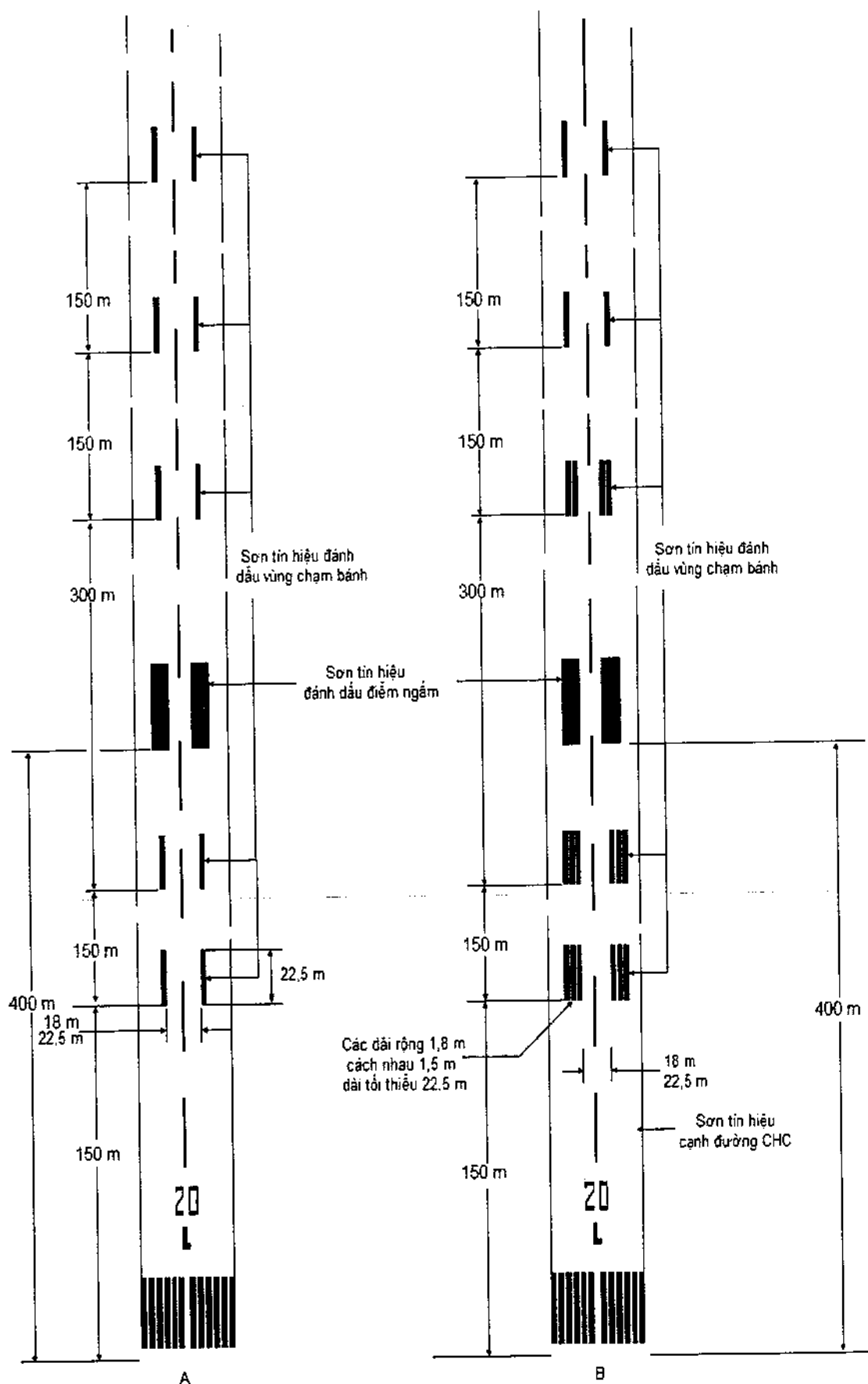
Hình 7 - Sơn tín hiệu đánh dấu điểm ngắm và vùng chạm bánh (minh họa cho đường CHC có chiều dài từ 2400 m trở lên)
