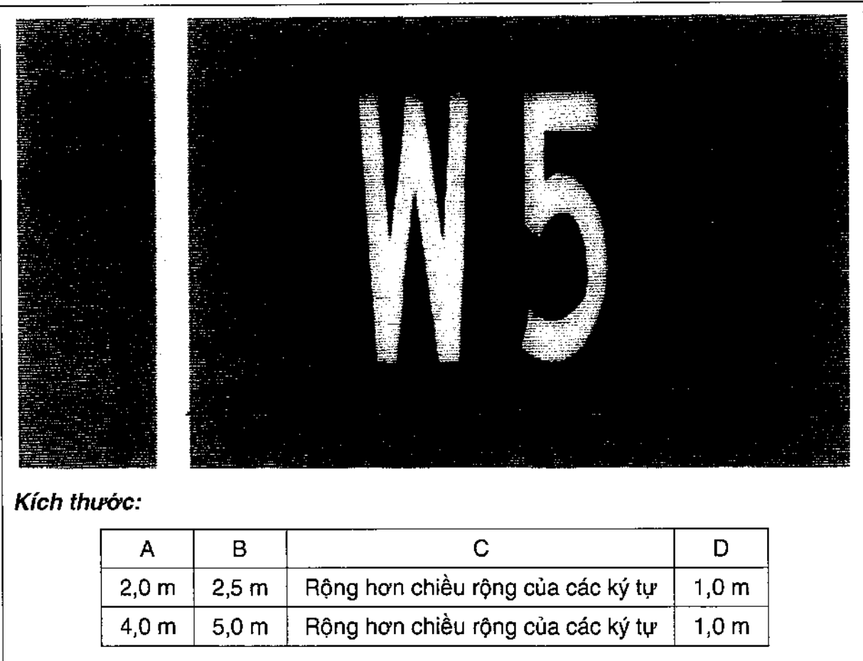
Hình 25 – Sơn tín hiệu biển báo vị trí
