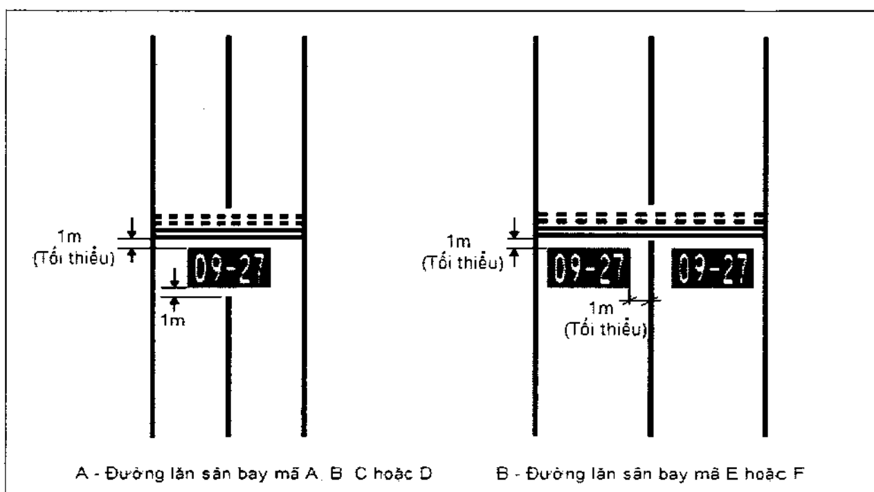
Hình 23 - Sơn tín hiệu chỉ dẫn bắt buộc
