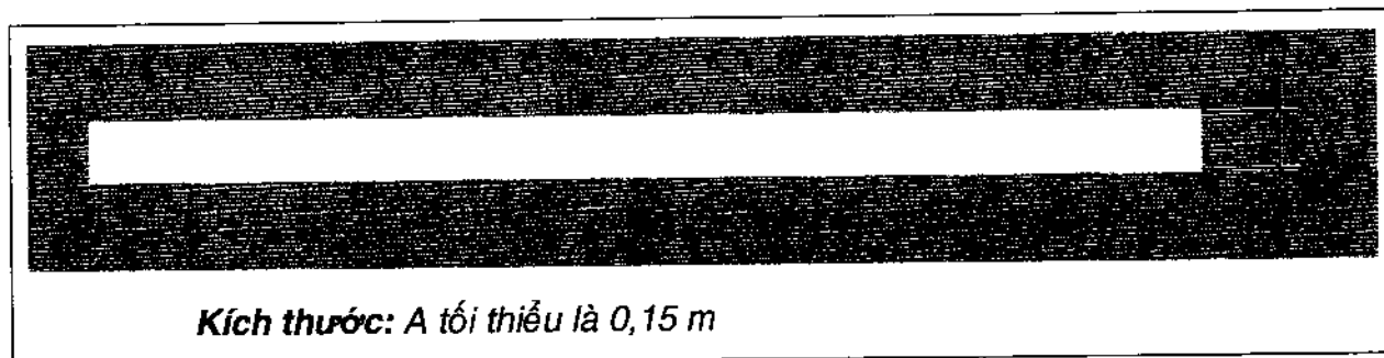
Hình 9 – Hình dạng, kích thước của sơn tín hiệu đường tìm đường lăn, sơn tín hiệu sân quay đầu đường CHC
