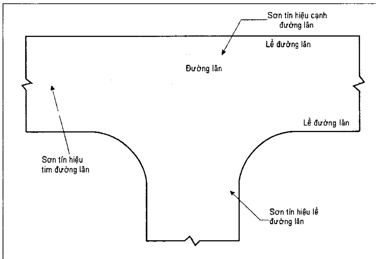
Hình 21 - Sơn tín hiệu lề đường làn (Tại nơi đường làn giao với đường làn)
