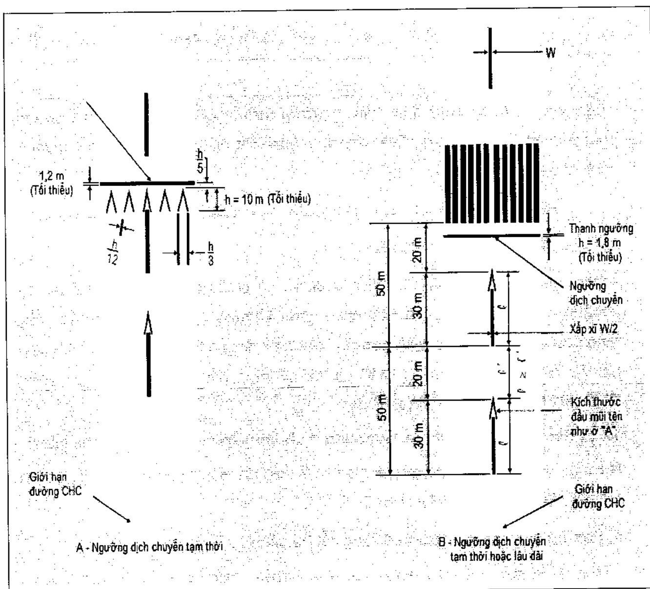
Hình 3 - Sơn tín hiệu đánh dấu ngưỡng đường CHC bị dịch chuyển
