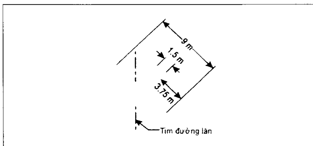
Hình 22 - Sơn tín hiệu đóng cửa đường lán
