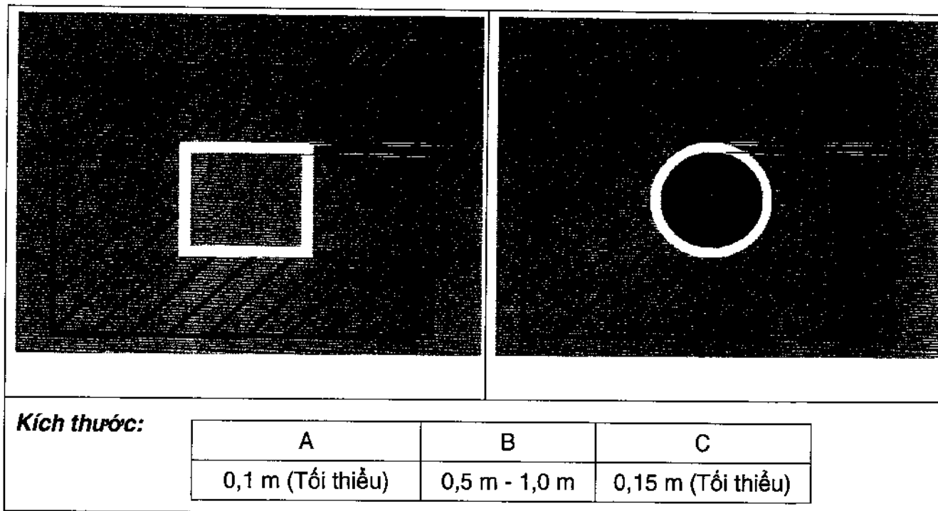
Hình 44 - Sơn tín hiệu khu vực giới hạn di chuyển cầu hành khách
