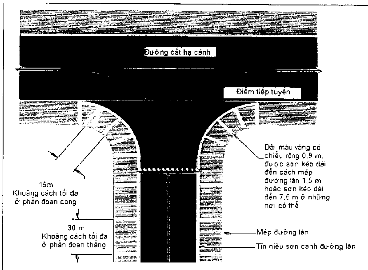
Hình 20 - Sơn tín hiệu lề đường làn (Tại nơi đường làn giao với đường CHC)
