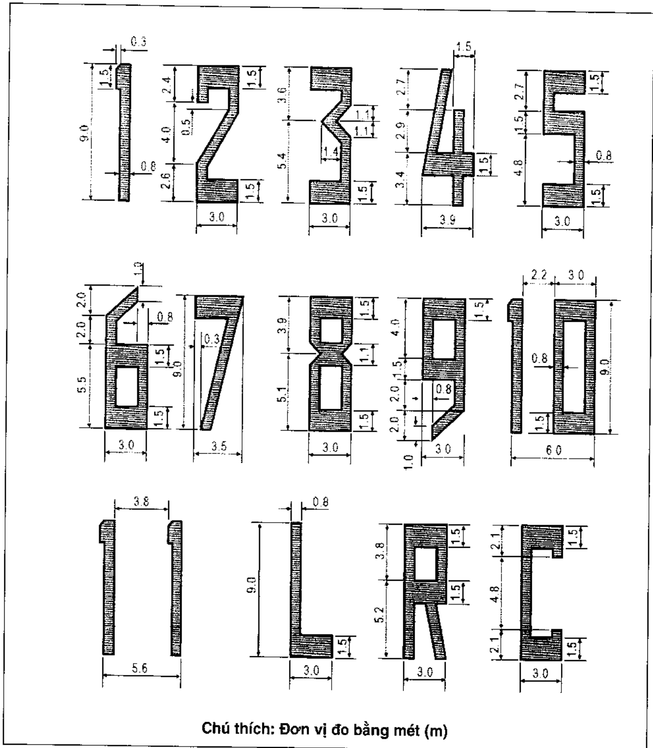
Hình 2 - Hình dạng, tỷ lệ chữ và số chỉ hướng đường cắt hạ cánh
