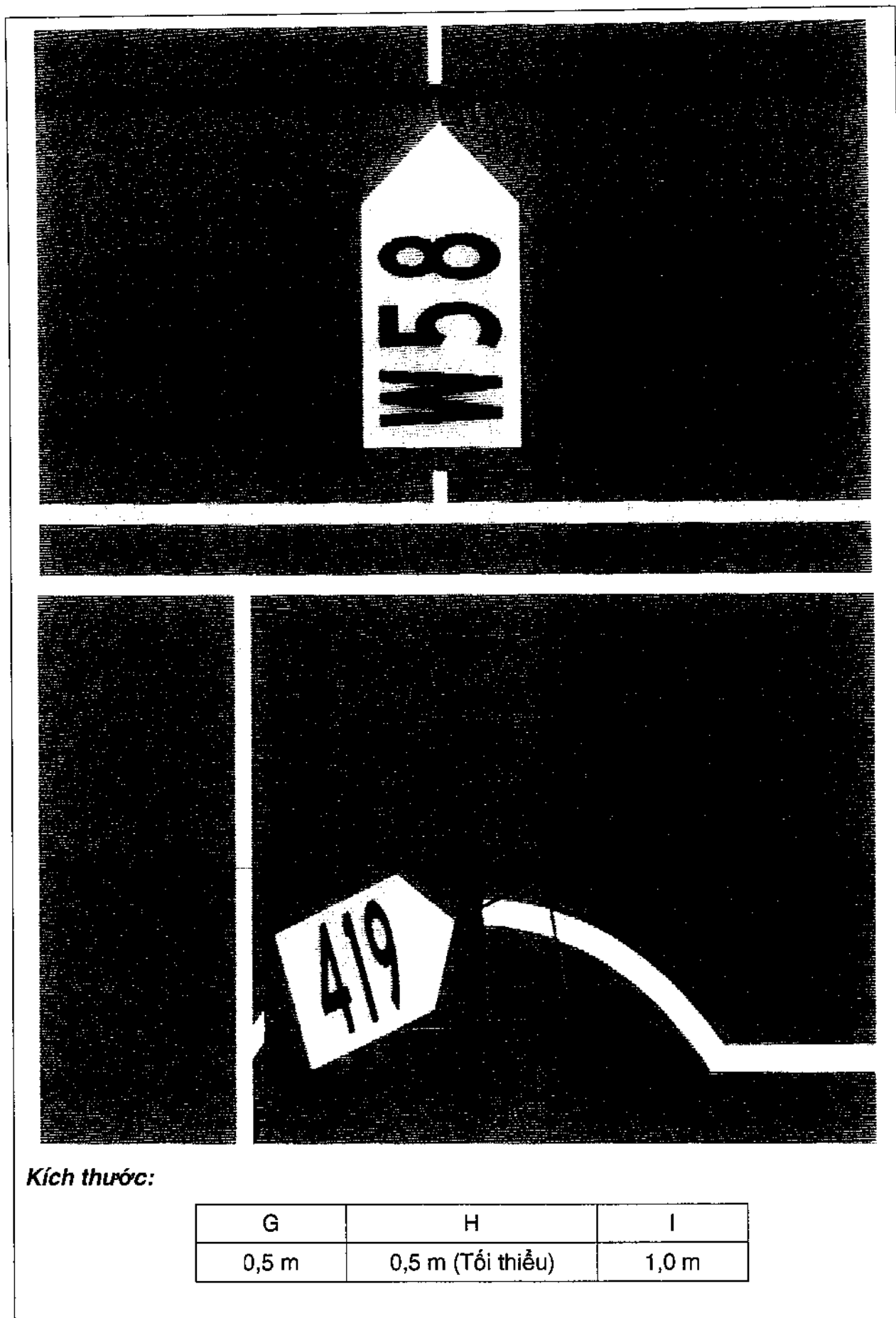
Hình 33 - Sơn tín hiệu nhận dạng đến vị trí đỗ tàu bay (Góc 61 0 đến 90 0 )
