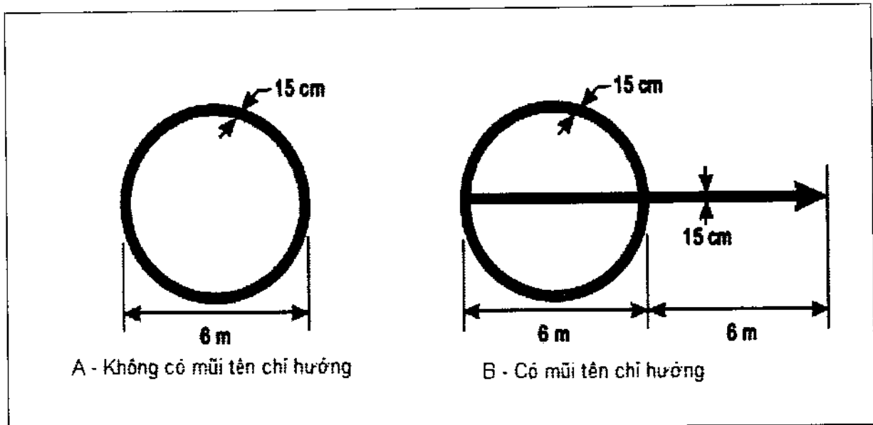
Hình 49 - Sơ đồ tín hiệu đánh dấu điểm kiểm tra đài VOR
