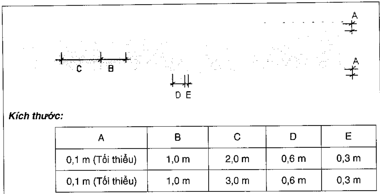
Hình 46 - Sơn tín hiệu đường công vụ cho các phương tiện mặt đất
