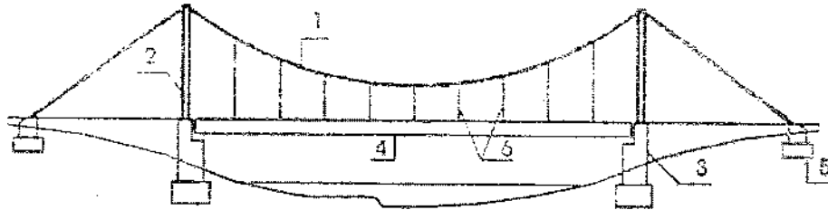
Hình 1: Sơ đồ cấu tạo cầu treo dân sinh một nhịp
