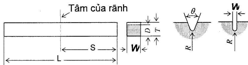
Hình 6A/2.1 - Mẫu thử độ dai va đập
