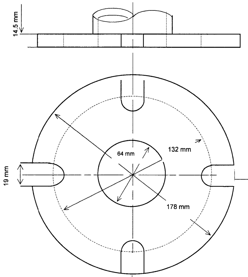
Hình 5/4.10 - Đầu nối bờ tiêu chuẩn
