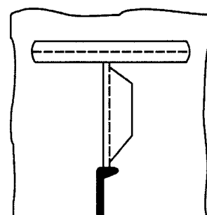
Hình 2A/2.3.2-5. Hàn mã với nẹp gia cường nằm trong mặt phẳng vuông góc với mặt phẳng của các mã
