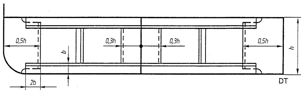
Hình 2A/2.4.3 - Kết cấu đà ngang hờ
