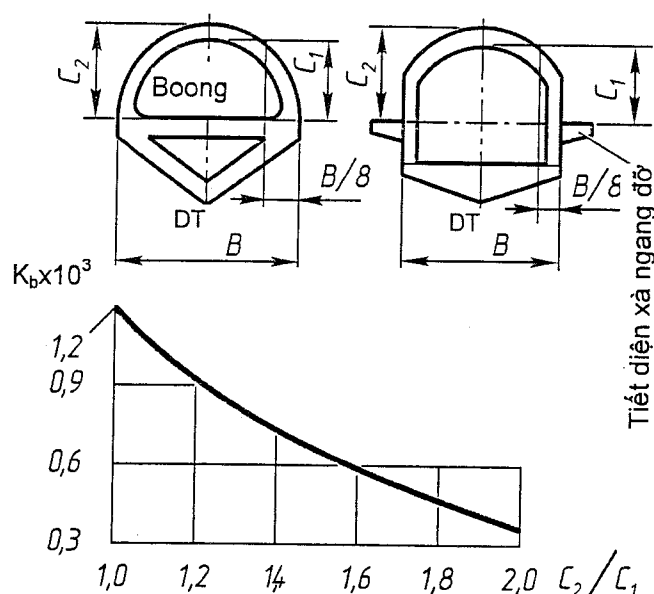
Hình 2A/6.3.5 - Hệ số k_b
