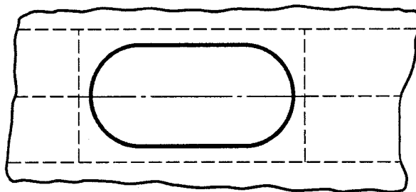
Hình 2A/2.3.3-1. Các cơ cấu gia cường ở lỗ khoét
