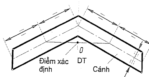
Hình 2A/6.2.3-1 - Điểm đặt lực nâng ở cánh mũi
