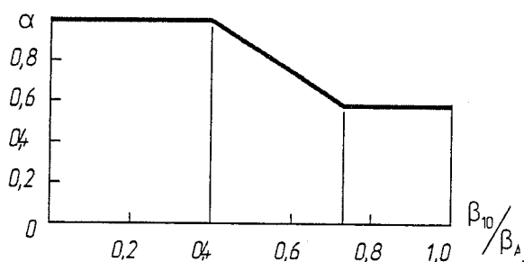
Hình 2A/6.3.1-2 - Hệ số \alpha
