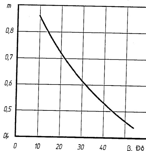
Hình 2A/6.2.3-2 - Đồ thị mối liên hệ của hệ số m với góc cắt ngang tính toán của đáy tàu \beta
