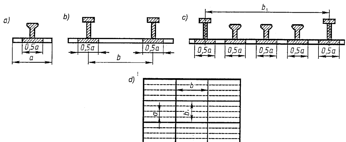
Hình 2A/4.3.2-1 - Chiều rộng mép kèm
