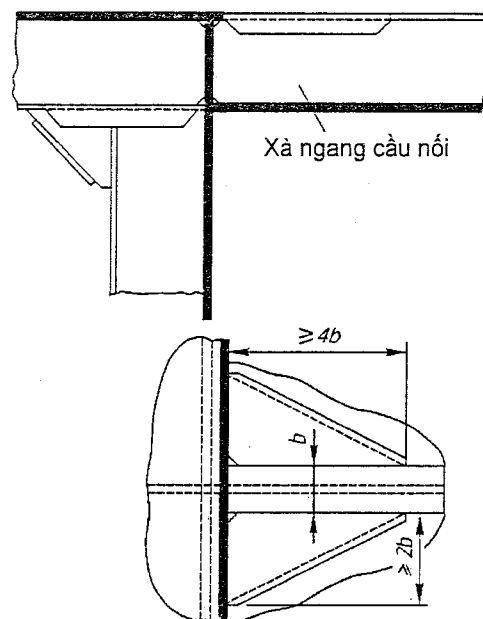
Hình 2A/5.4.12-2 - Liên kết mép xà khỏe của cầu nổi hờ ở phía trên với boong
