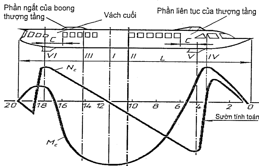
Hình 2A/6.1.2 - Biểu đồ M_c và N_c cho tàu cánh ngầm
