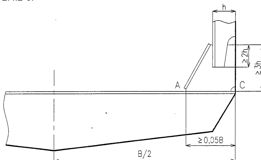
Hình 2A/2.4.2 - Quy cách mã hông
