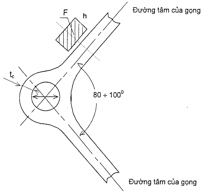
Hình 2A/2.4.10-3 - Giá đỡ trực chân vịt
