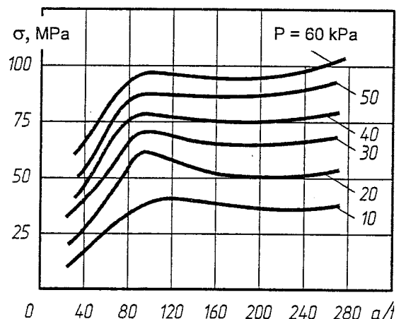
Hình 2A/4.3.6-2 - Đồ thị xác định ứng suất tại mặt cắt của đế không được tiêu chuẩn hoá, ứng suất \sigma do tác động của tải trọng ngang
