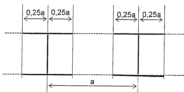
Hình 2A/3.1.2-2 - Các kết cấu dọc của đáy dưới tham gia vào tổng diện tích
