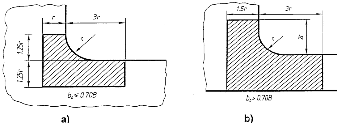
Hình 2A/2.4.5 - Phần boong không được bố trí đường hàn giáp mối và khoét lỗ
