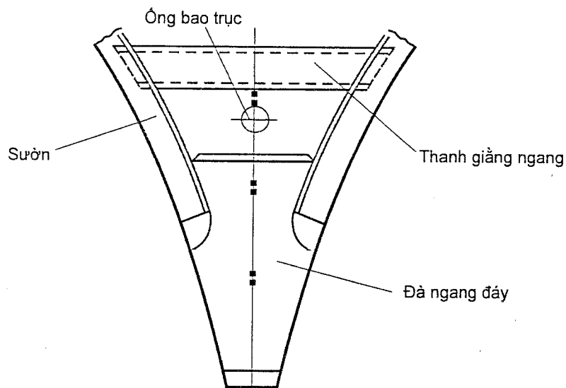
Hình 2A/2.4.9 - Liên kết thanh giằng
