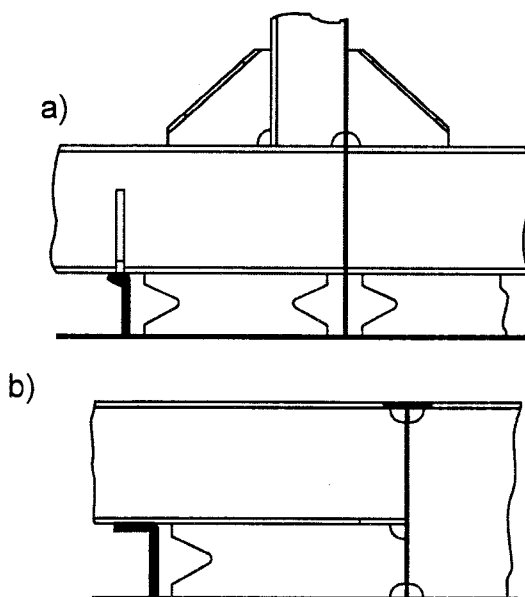
Hình 2A/2.3.2-2. Kết cấu hệ thống kiểu treo
