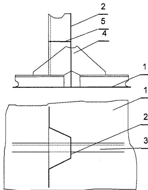
Hình 2A/2.3.4-2. Vị trí bố trí nẹp
