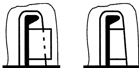
Hình 2A/2.3.2-1 Liên kết cơ cấu thường và cơ cấu khỏe không kín nước (vách không kín nước)
