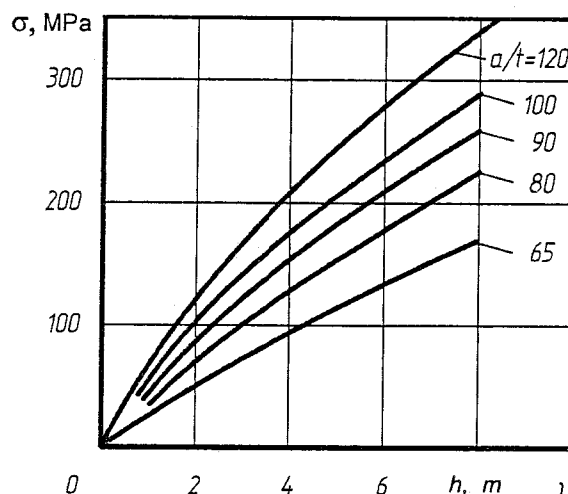
Hình 2A/4.3.6-1 - Đồ thị xác định ứng suất lớn nhất \sigma tại tiết diện mặt cắt đế tựa của tấm ngàm cứng chịu kéo tác động của tải trọng ngang
