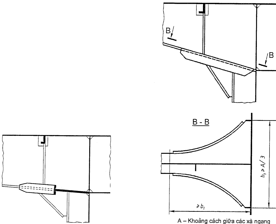
Hình 2A/5.4.9-1 - Bố trí sống dọc ở sàn dưới của cầu nổi
