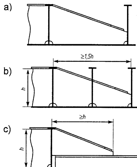
Hình 2A/2.3.1-2. Kết cấu chỗ kết thúc dầm khỏe
