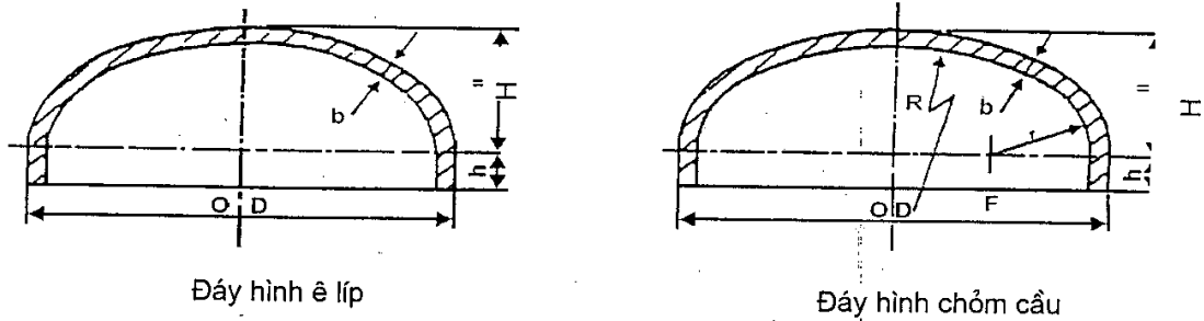
Hình 19a. Hình dạng các đáy bình
