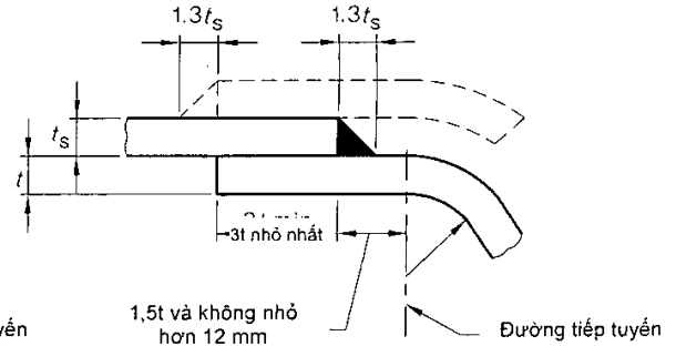
h) Ống hàn đơn
