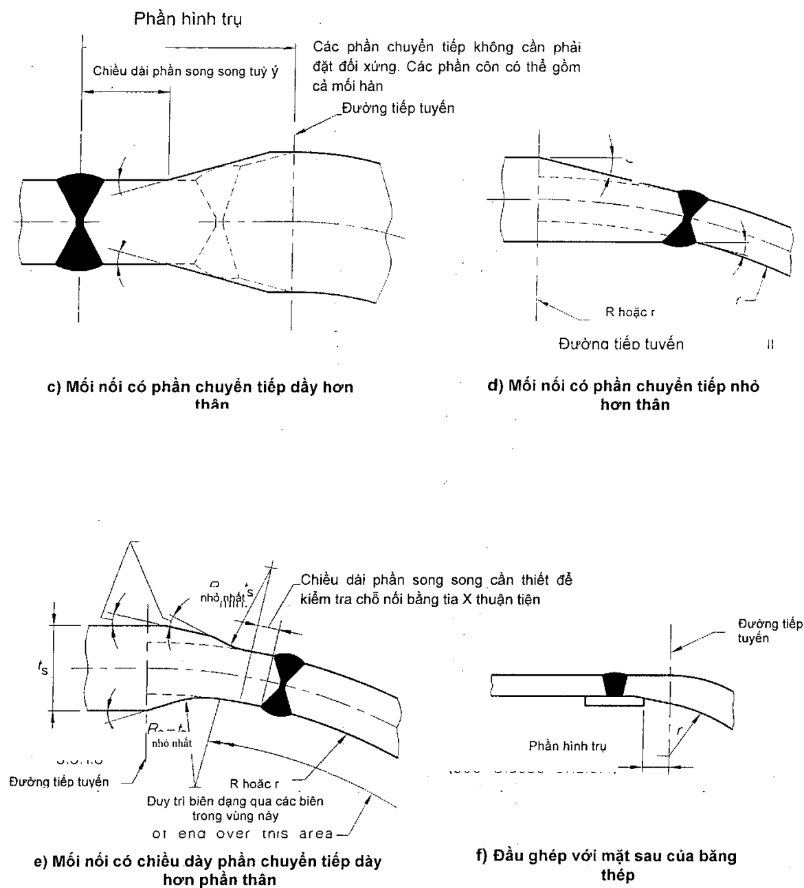
Hình 6. Mối ghép của các ống cong (tiếp theo)
