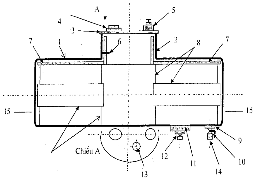
Hình 12. Cấu tạo chung của xi téc
