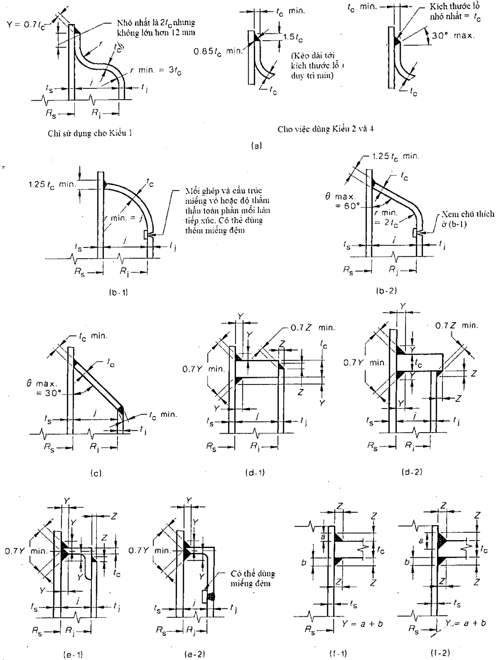
Hình 9. Một số kiểu vãnh chặn vò được chấp nhận
