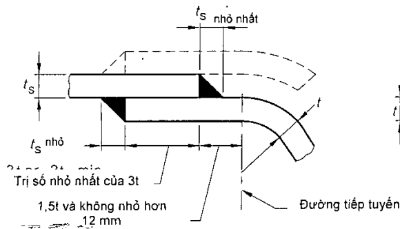
g) Cặp ống hàn
