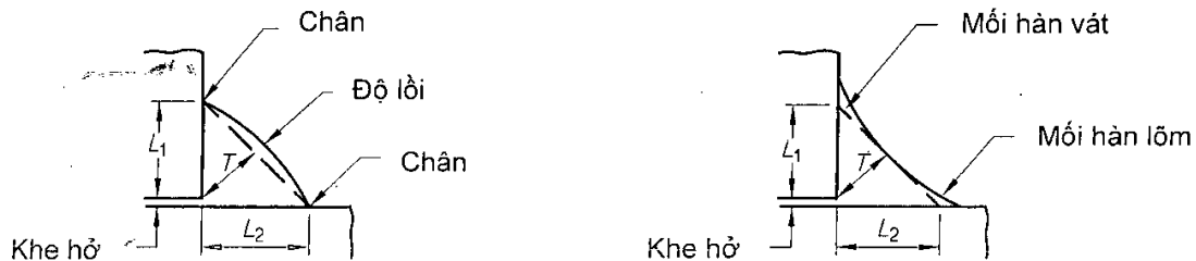
a) Mối hàn góc lồi
