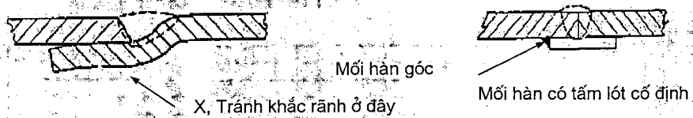
Hình 18a. Các kiểu mối hàn giáp mép dọc
