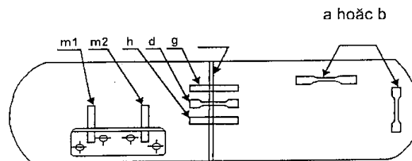
Hình 14b. Bình chứa chỉ có các mối hàn theo chu vi và cụm van lắp bên cạnh - vị trí lấy các mẫu thử
