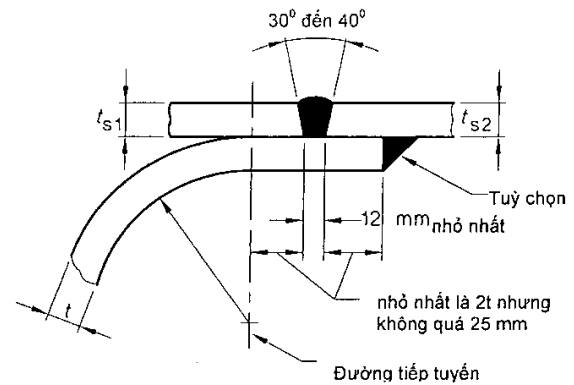
k) Đoạn chuyển tiếp của đáy
