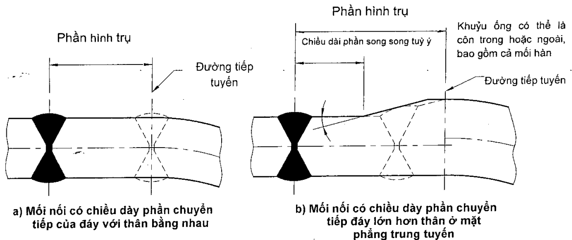
Hình 6. Mối ghép của các đáy cong
