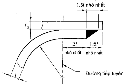
j) Ống hàn đơn
