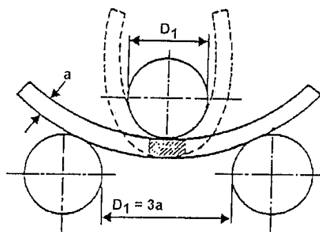
Hình 15a. Minh họa phép thử uốn
