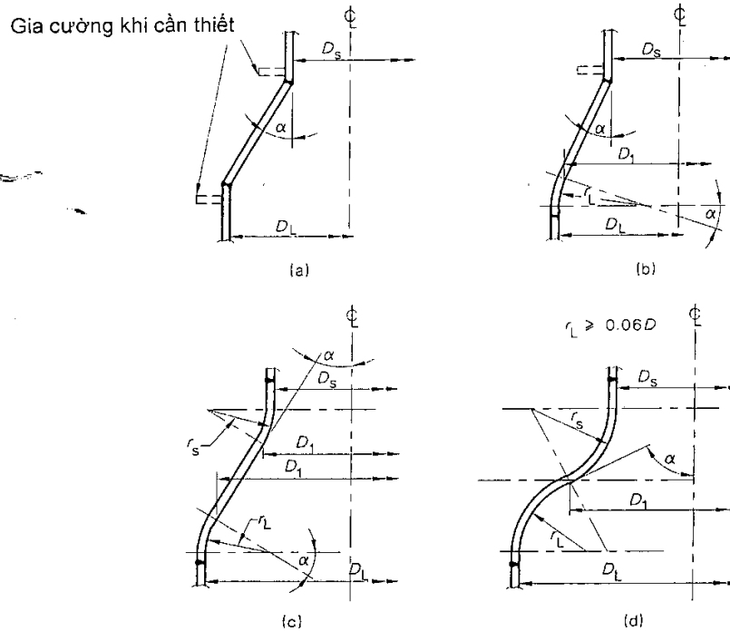
Hình 4. Đáy côn và đoạn côn
