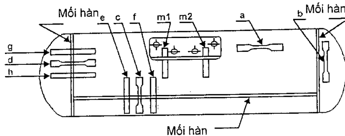
Hình 14a. Bình chứa có các mối hàn dọc và theo chu vi - vị trí lấy các mẫu thử
