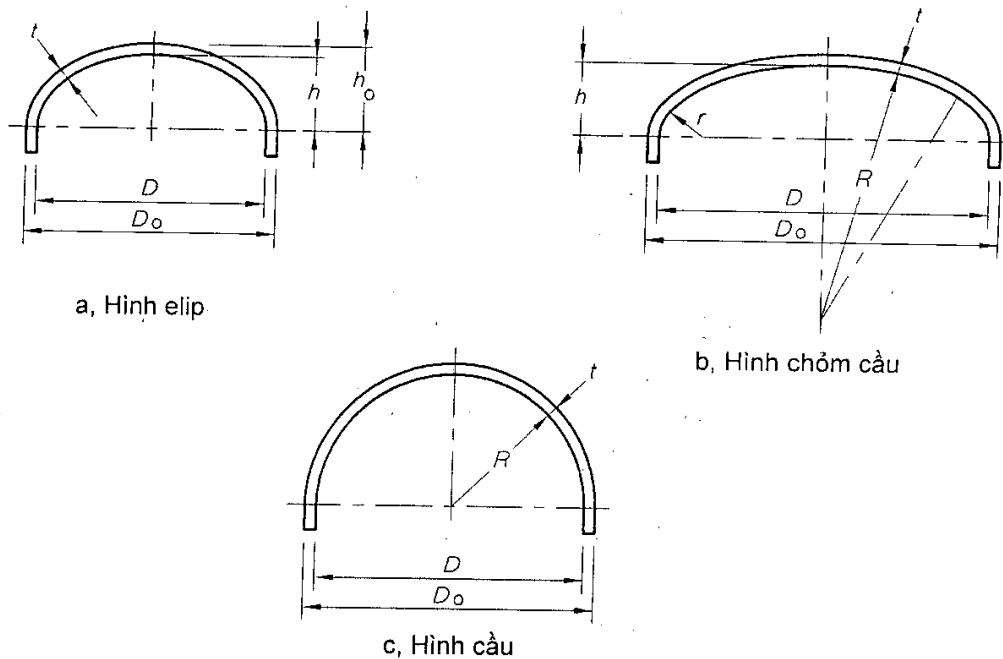
Hình 5. Kích thước của các dáy
