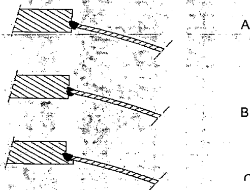
Hình 18c. Các thí dụ về các tấm được hàn nổi
