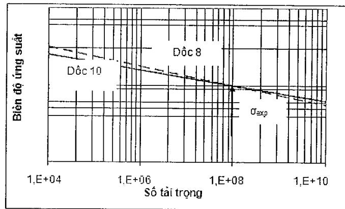
Hình 8G/5.9 Đường cong S-N dốc không đổi
