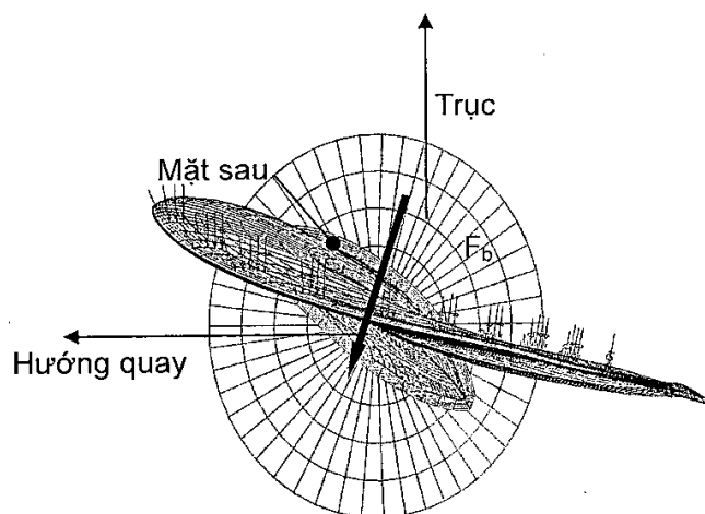
Hình 8G/5.5 Hướng của lực tác động lên cánh chân vịt
