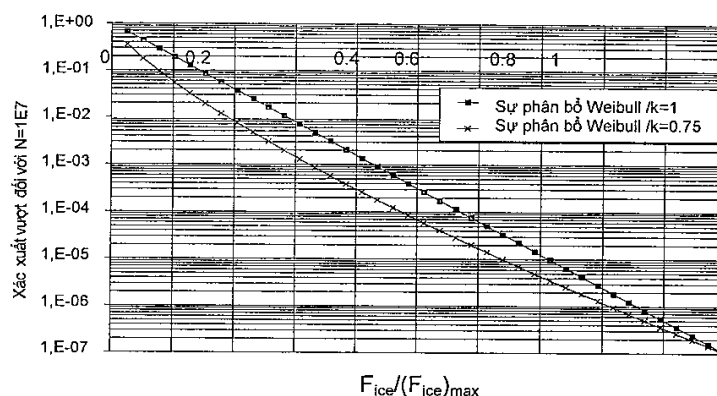
Hình 8G/5.6 Sử dụng phân bố Weibull (xác suất F_{ice} vượt (F_{ice})_{max} ) được sử dụng trong việc thiết kế mối
