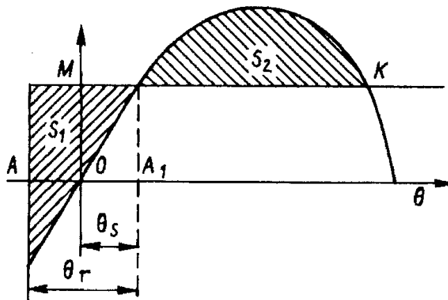
Hình 10/Phụ lục 1/1.2.2 Xác định mô men lật của cần cầu nổi ở trạng thái chằng giữ khi đi biển theo đường cong ổn định tĩnh
