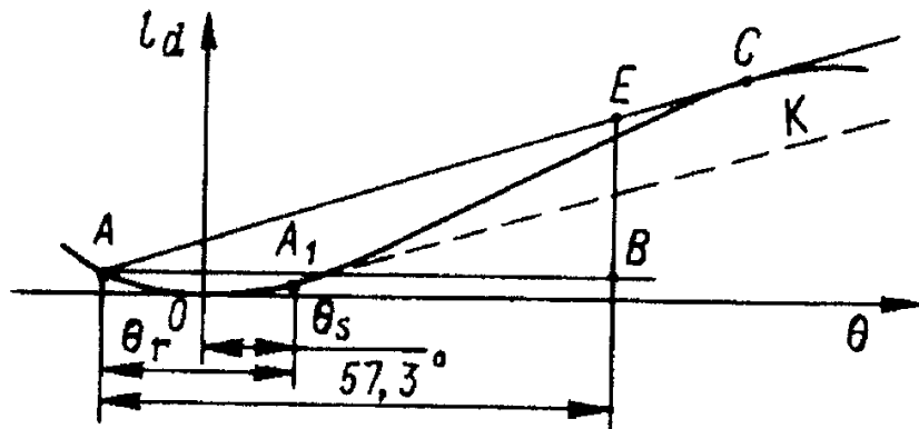
Hình 10/Phụ lục 1/1.2.1 Xác định mô men lật của cần cầu nổi ở trạng thái chằng giữ khi đi biển theo đường cong ổn định động.
