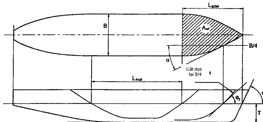
Hình 8G/5.4 Các kích thước
