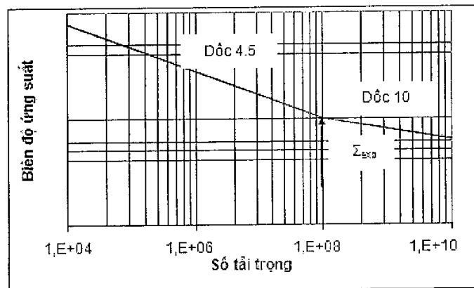
Hình 8G/5.8 Đường cong S-N hai dốc
