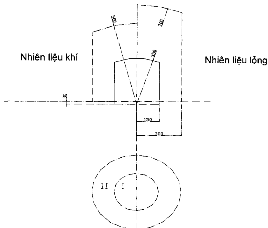
Hình 5: Lắp đặt thiết bị nấu nướng với ngọn lửa hở Các kích thước tính bằng (mm).
