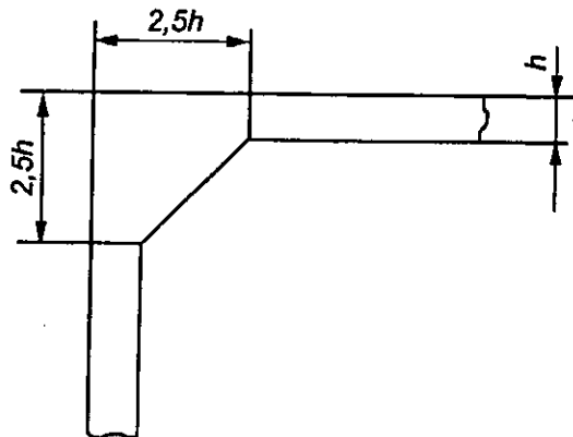
Hình 5 - Liên kết sườn và xà ngang boong
