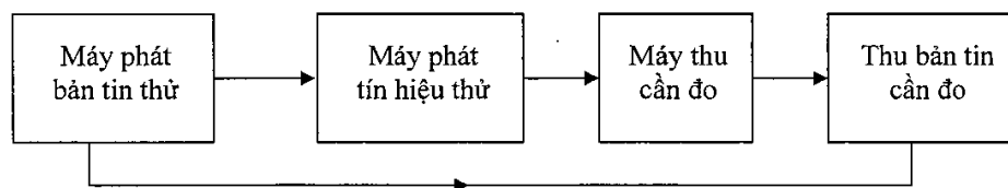
Hình 17 - Sơ đồ đo độ nhảy thu tại kênh 25 kHz
