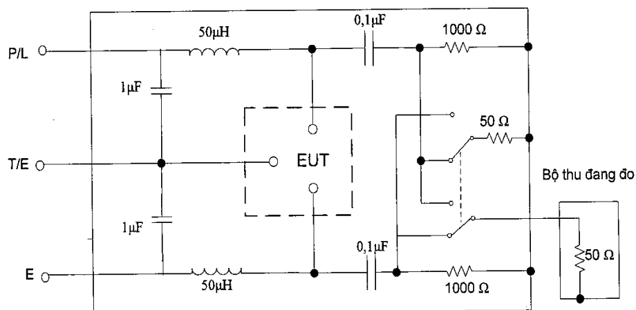
Hình 4b - Ví dụ mô phỏng mạng nguồn giả V 50 \Omega/50 \mu\text{H} để dùng trong dải tần 150 kHz tới 30 MHz
