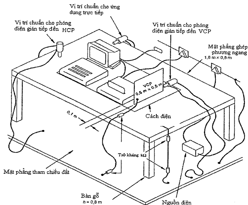
Hình 14 - Ví dụ thiết lập thiết bị đặt trên bàn cho phép thử miễn nhiễm phóng tĩnh điện (ESD) chỉ rõ vị trí cơ bản của thiết bị phát ESD
