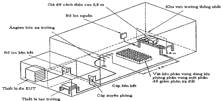
Hình 9 - Ví dụ điều kiện thử nghiệm thích hợp miễn nhiệm đối với tần số vô tuyến phân tán
