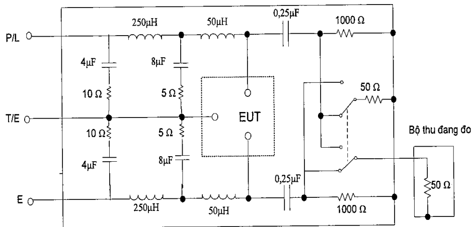
Hình 4a - Ví dụ mô phỏng mạng nguồn giả V 50 \Omega/50 \mu\text{H} + 5 \Omega để dùng trong dải tần 10 kHz tới 150 kHz
