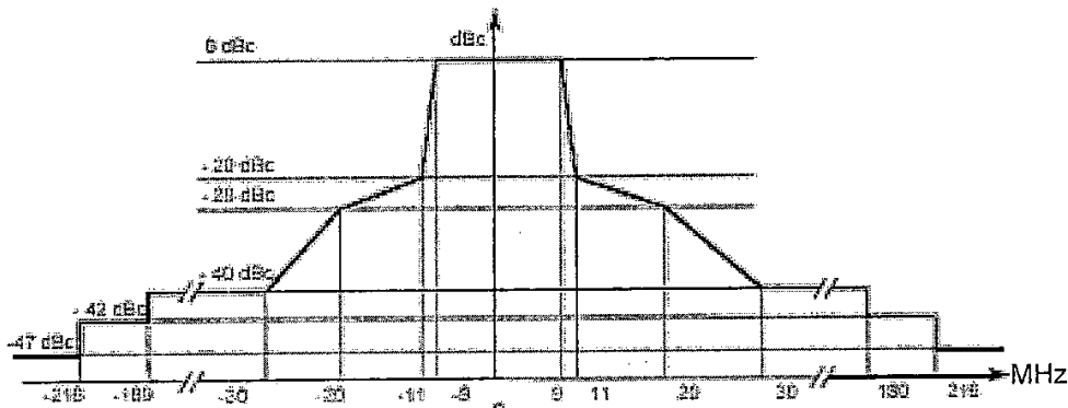
Hình 1 - Mặt nạ công suất phổ phát
