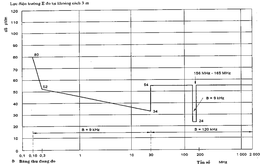
Hình 6 - Giới hạn phát xạ bức xạ từ các cổng vô
