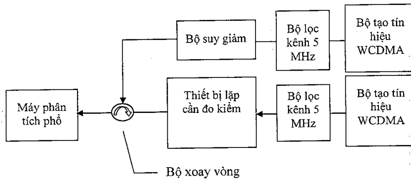
Hình D.6 – Sơ đồ hệ đo xuyên điều chế đầu ra
