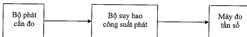
Hình 15 - Sơ đồ đo lỗi tần số
