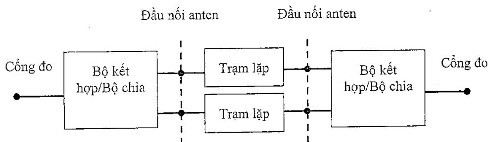
Hình A.1 - Ví dụ về cấu hình thiết bị lắp.
