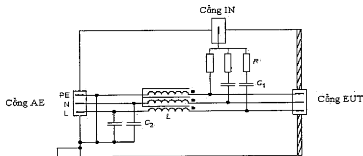
Hình 7 - Sơ đồ thiết lập thử miễn nhiễm đối với nhiễu dẫn tần số vô tuyến
