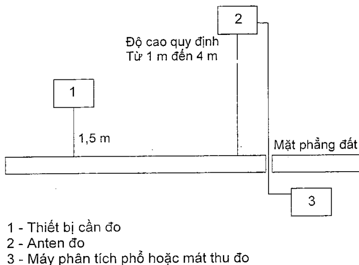
Hình B.1 – Bố trí phép đo 1
