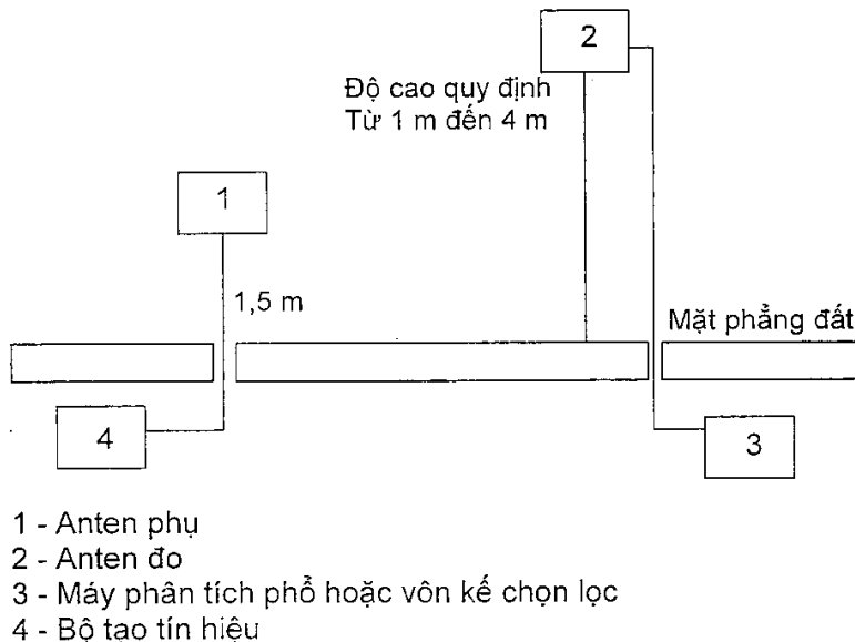
Hình B.2 – Bố trí phép đo 2
