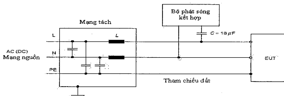
Hình 11a - Ví dụ thiết lập phép thử ghép điện dung trên đường AC/DC; ghép đường tới đường, đầu ra thiết bị phát thả nổi
