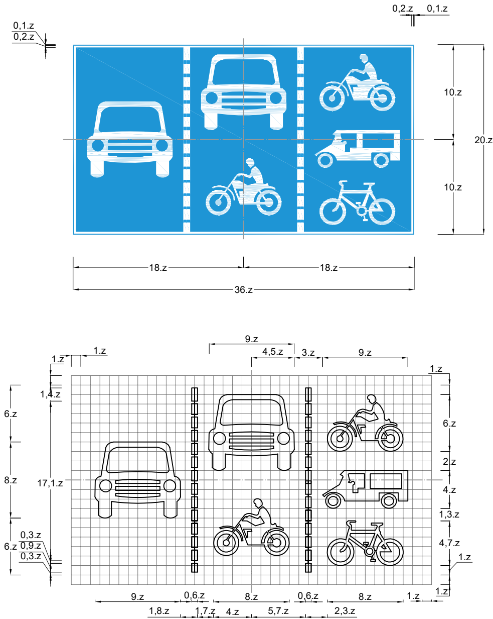
Biển số R.415a: Biển gộp làn đường theo phương tiện
