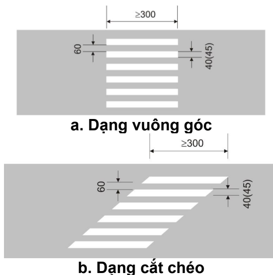
Hình G.51 - Vạch đi bộ qua đường – Mẫu 1
