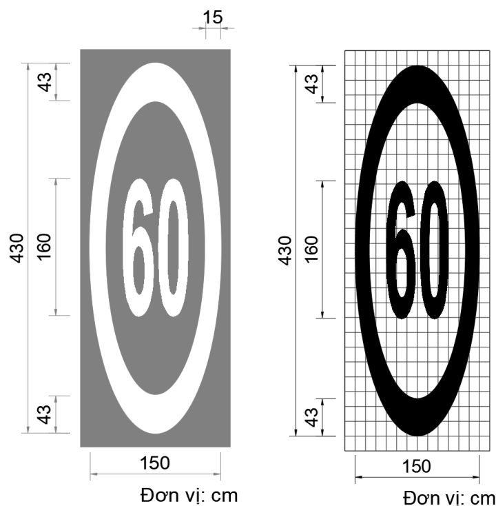
Hình G.85 - Vạch sơn tốc độ tối đa cho phép trên mặt đường áp dụng cho đường có tốc độ xe chạy <80 km/h
