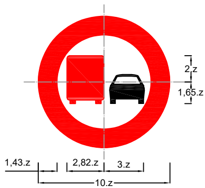
Biển số P.126: Cấm ô tô tải vượt
