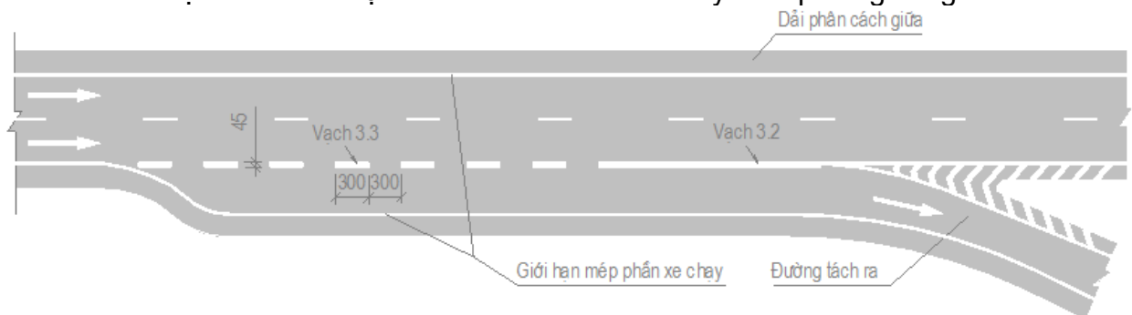
Hình G.15 - Minh họa bố trí vạch sơn khu vực tách làn kiểu song song
