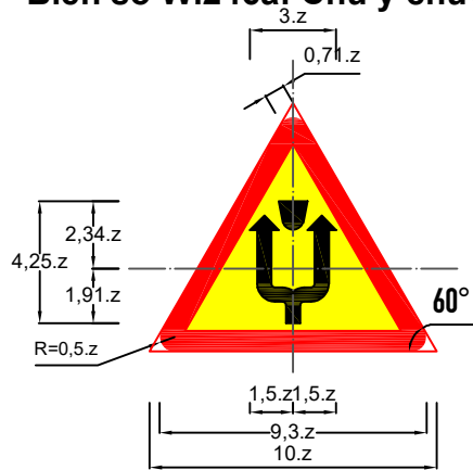
Biển số W.246a: Chú ý chướng ngại vật - Vòng tránh ra hai bên
