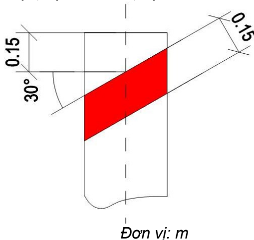
Hình G.67 - Chi tiết vạch 8.4
