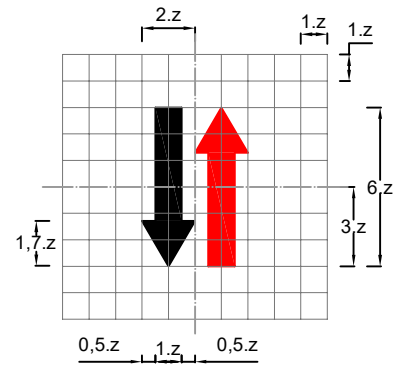
Biển số P.132: Nhường đường cho xe cơ giới đi ngược chiều qua đường hẹp
