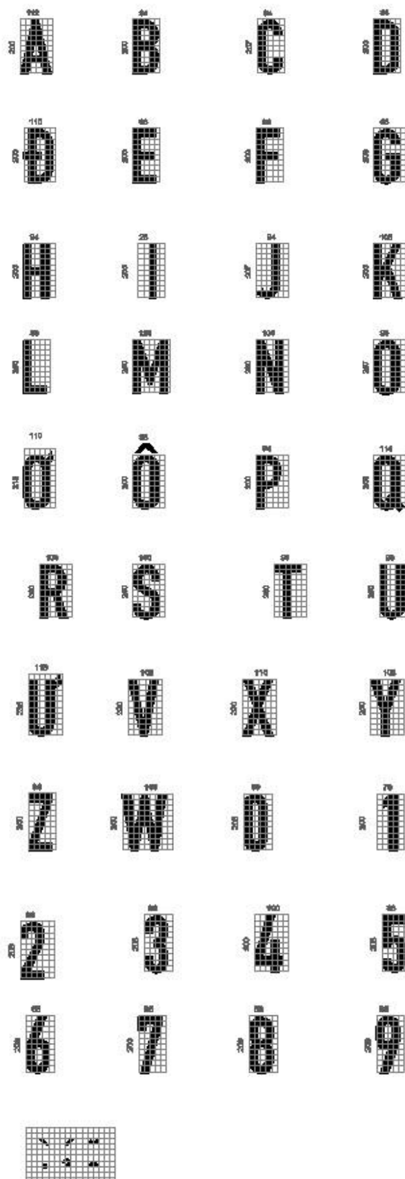
Ghi chú: đơn vị mm Hình K.4 - Chi tiết chữ viết và con số dạng chữ in hoa, kiểu chữ nén (gt1)
