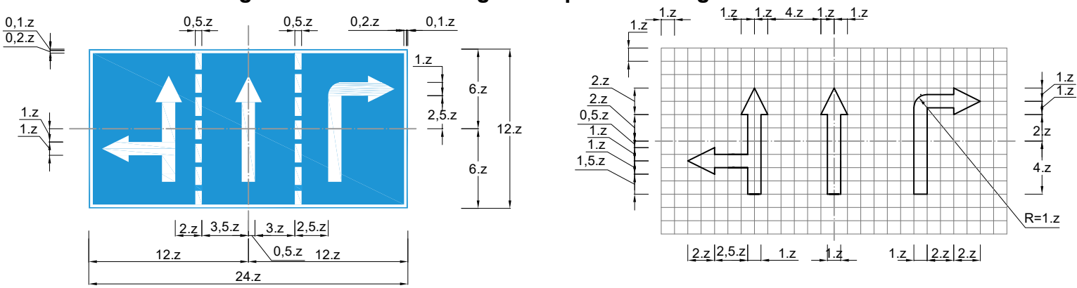
Biển số R.411: Hướng đi trên mỗi làn đường theo vạch kẻ đường
