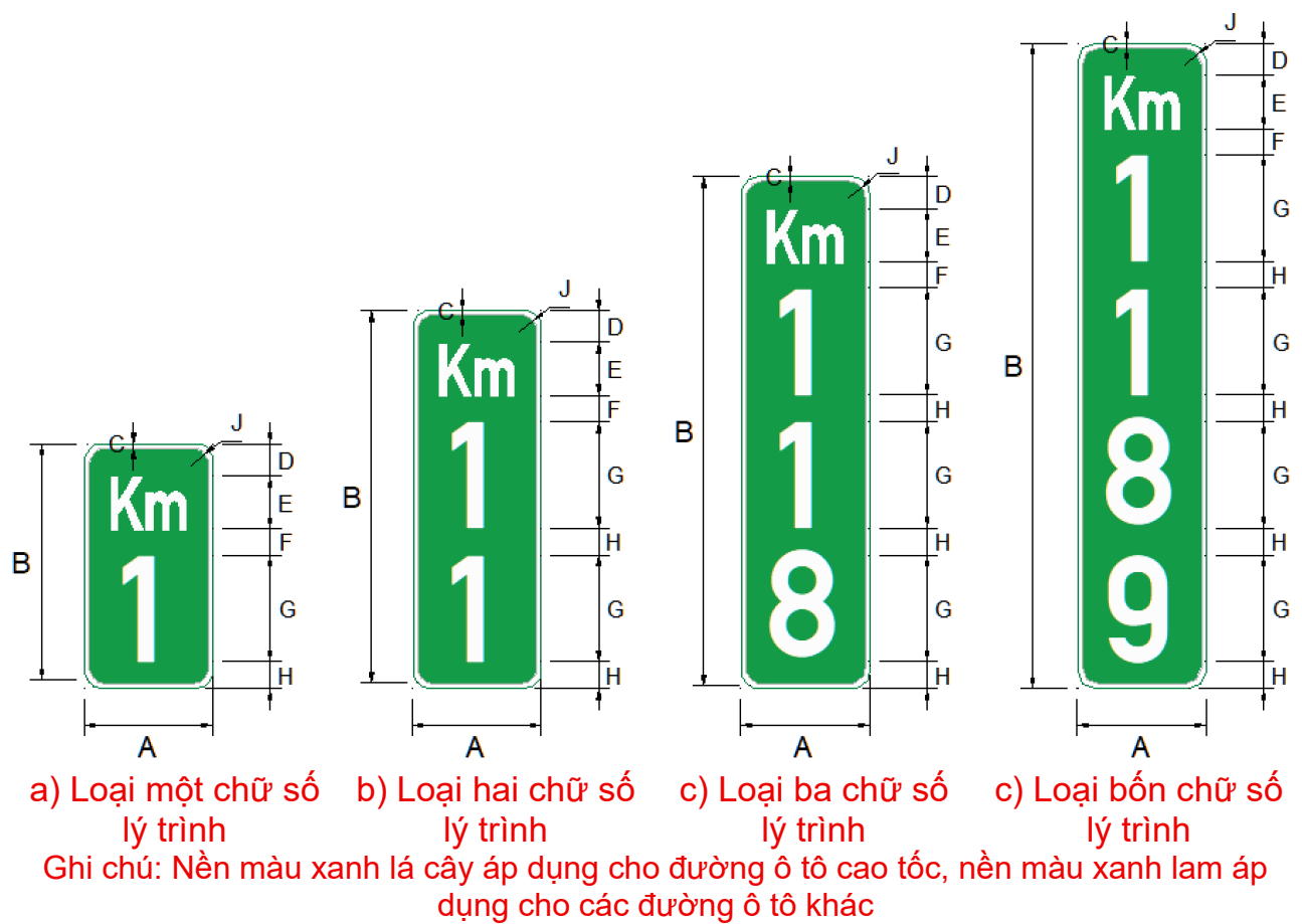
Hình I.3 – Cột kilômét dạng tấm hình chữ nhật đặt ở lề đường Bảng các giá trị kích thước trên Hình I.3
