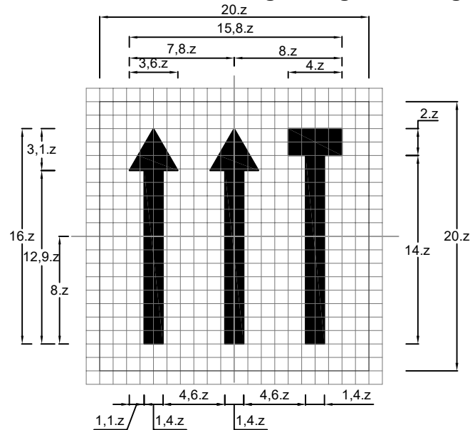
Biển số S.H,6 : Ngoại lệ
