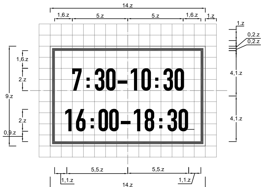
Biển số S.508b : Biểu thị thời gian
