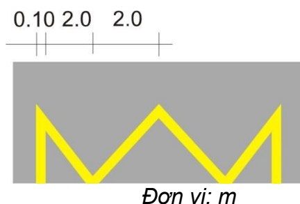
Hình G.72 - Chi tiết vạch số 9.2
