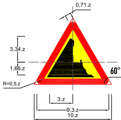
Biển số W.223a: Vách núi nguy hiểm
