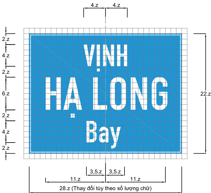
Biển số I.422b : Di tích lịch sử
