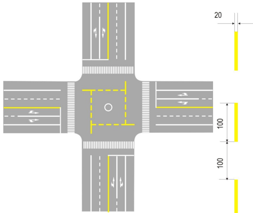
Hình G.54 - Vạch xác định khu vực cấm xe thô sơ trong nút giao
