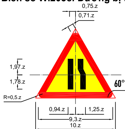
Biển số W.203c: Đường bị thu hẹp về phía phải
