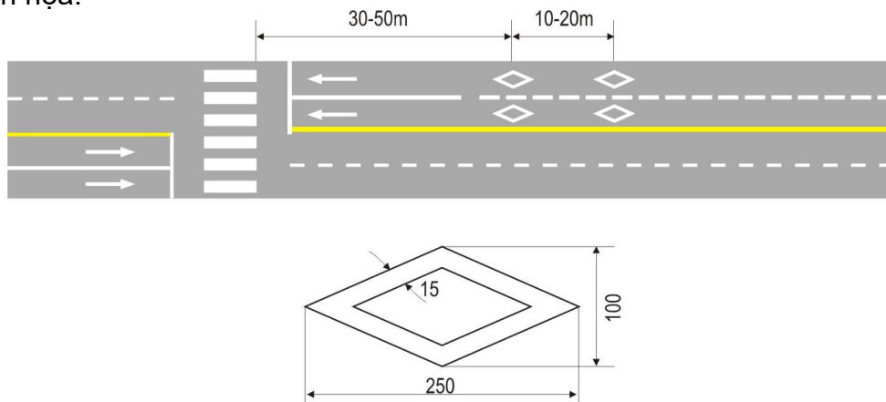
Hình G.55 - Vạch chỉ dẫn sắp đến chỗ có bố trí vạch đi bộ qua đường
