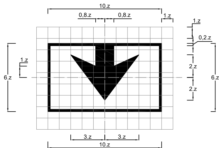
Biển số S.504 : Làn đường
