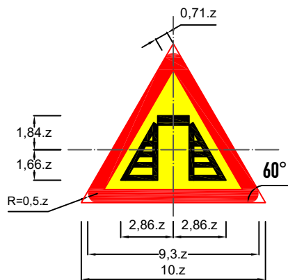
Biển số W.213: Cầu tạm
