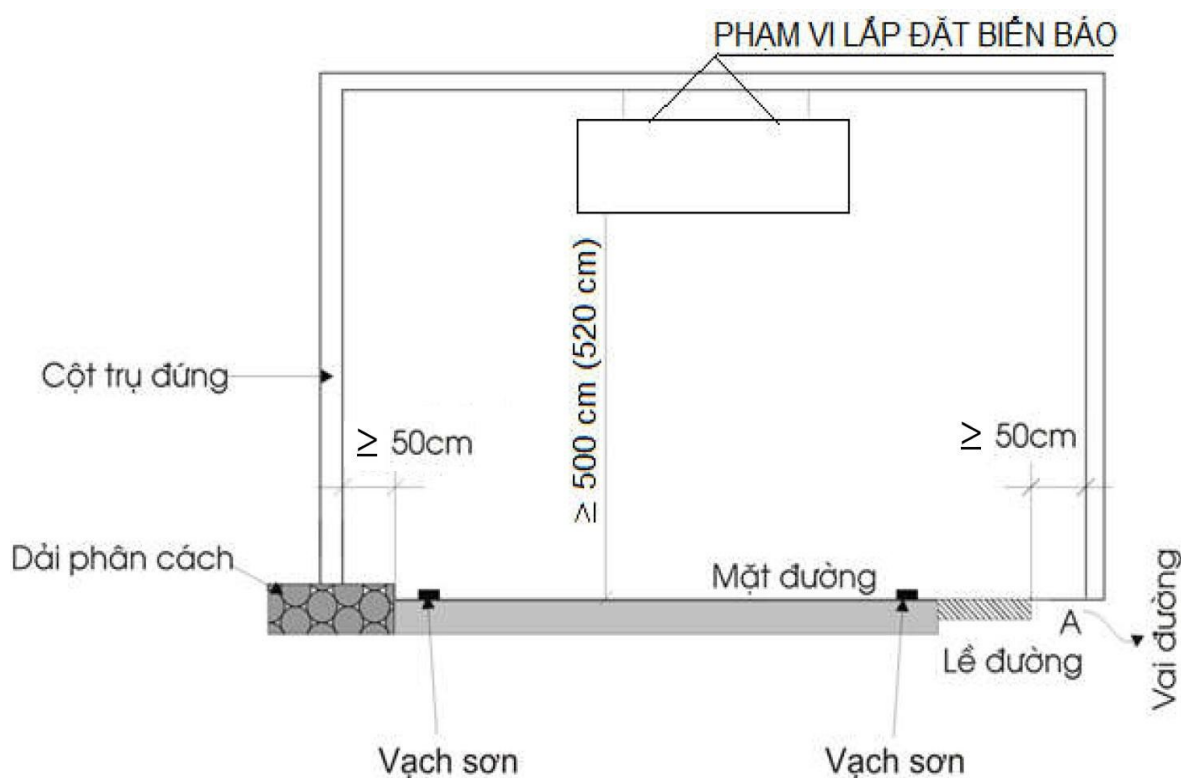
Hình 2 - Giá long môn
