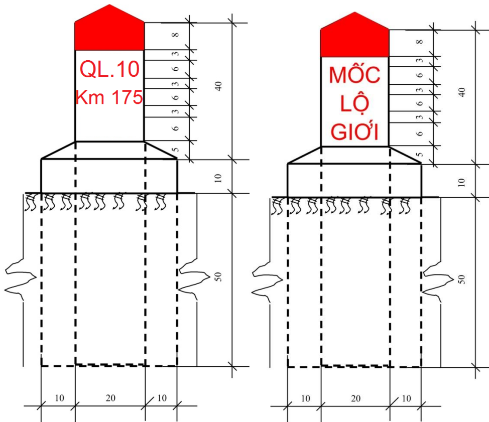
Hình I.4 - Cọc mốc lộ giới
