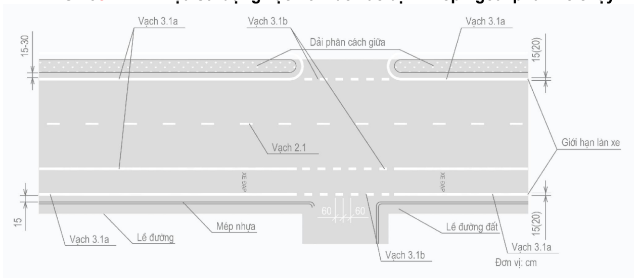
Hình G.13c - Minh họa sử dụng vạch 3.1 để xác định mép ngoài phần xe chạy
