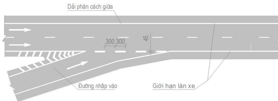
Hình G.16 - Minh họa bố trí vạch sơn khu vực nhập làn kiểu trực tiếp - Bố trí vạch sơn khu vực nhập làn kiểu có làn chuyển tiếp song song:
