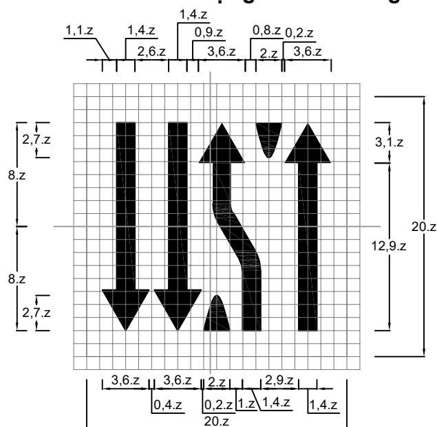
Biển số S.G,11c: Biển chỉ dẫn số lượng làn và hướng đi cho từng làn
