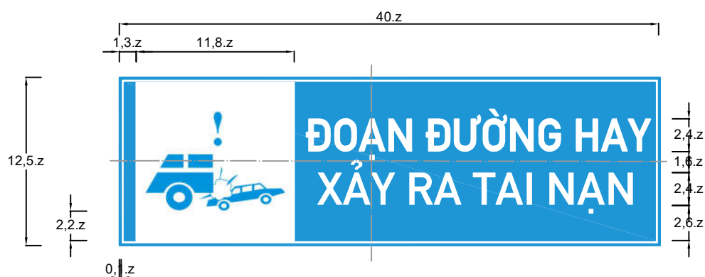
Biển số I.445g: Biển báo mô tả tình trạng đường
