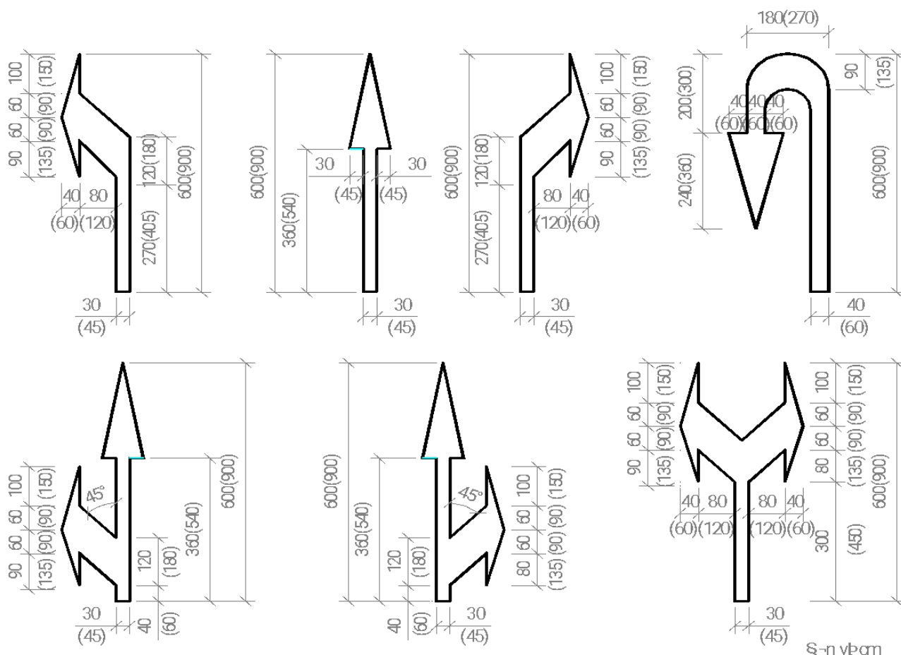
Hình G.74 - Kích thước của mũi tên chỉ đường áp dụng cho đường có tốc độ xe chạy cao
