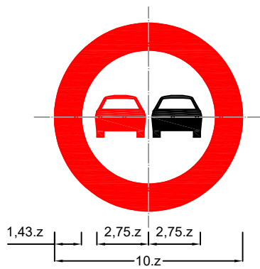
Biển số P.125: Cấm vượt
