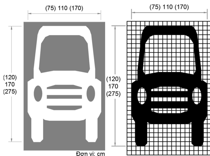
Hình G.84 - Vạch ký hiệu làn đường dành riêng cho ô tô
