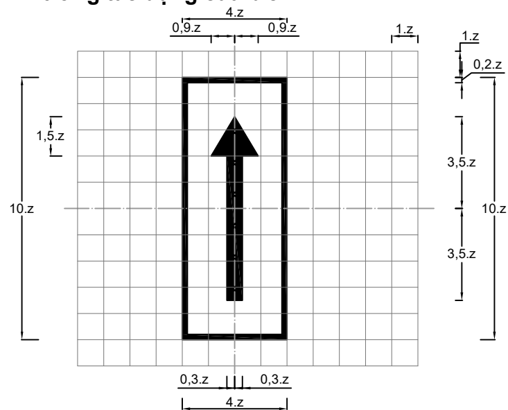
Biển SH.3a: Hướng tác dụng của biển
