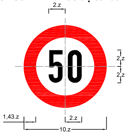
Biển số P.127: Tốc độ tối đa cho phép
