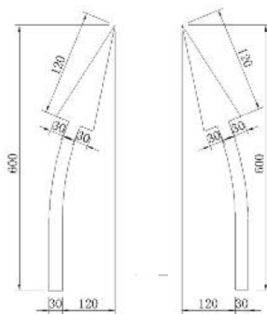
Hình G.76 - Kích thước vạch mũi tên báo số làn xe phía trước bị giảm e. Vạch 9.5: Vạch dạng chữ viết, chữ số, hoặc màu sắc trên mặt đường
