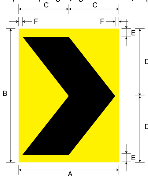
Hình 34b - Tiêu phản quang dạng mũi tên (bên trái) cho đường 2 chiều
