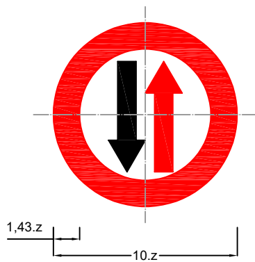
Biển số P.132: Nhường đường cho xe cơ giới đi ngược chiều qua đường hẹp
