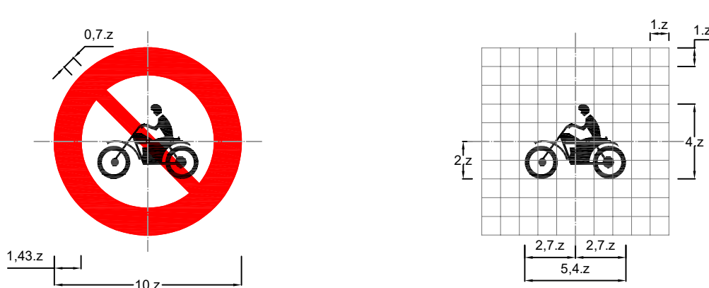
Biển số P.104: Cấm xe mô tô
