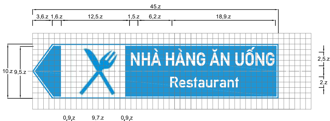
Biển số I.444l : Biển báo chỉ dẫn địa điểm
