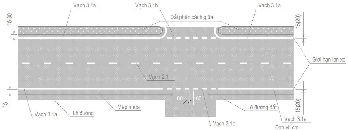
Hình G.13c - Minh họa sử dụng vạch 3.1 để xác định mép ngoài phần xe chạy
