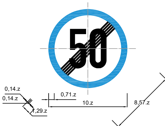
Biển DP.134: Hết hạn chế tốc độ tối đa
