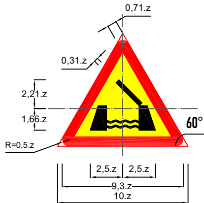
Biển số W.214: Cầu quay - cầu cắt
