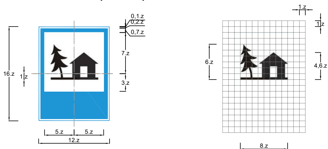
Biển số I.433e : Báo hiệu nhà trọ
