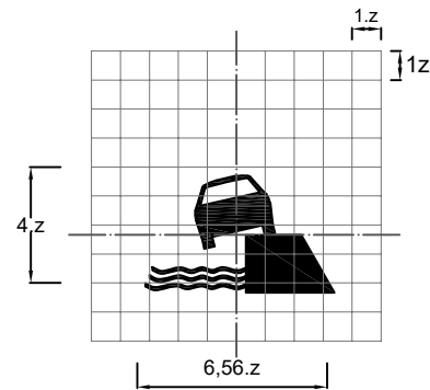
Biển số W.215c: Kè, vực sâu bên đường phía bên phải
