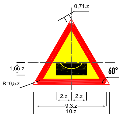
Biển số W.216a: Đường ngầm
