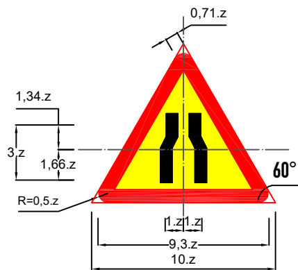
Biển số W.203a: Đường bị thu hẹp cả hai bên
