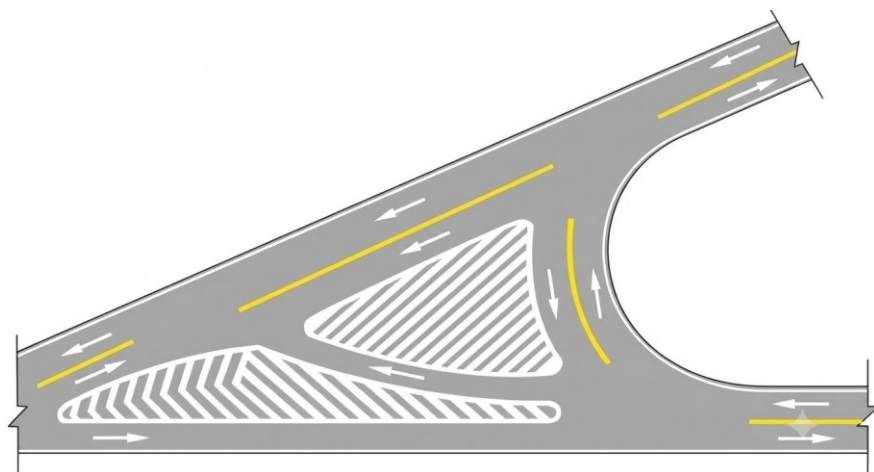
Hình G.33 - Bố trí vạch kênh hóa dòng xe ở ngã ba phức tạp – Mẫu 4
