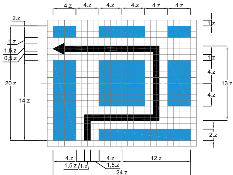
Biển số I.419a : Chỉ dẫn địa giới
