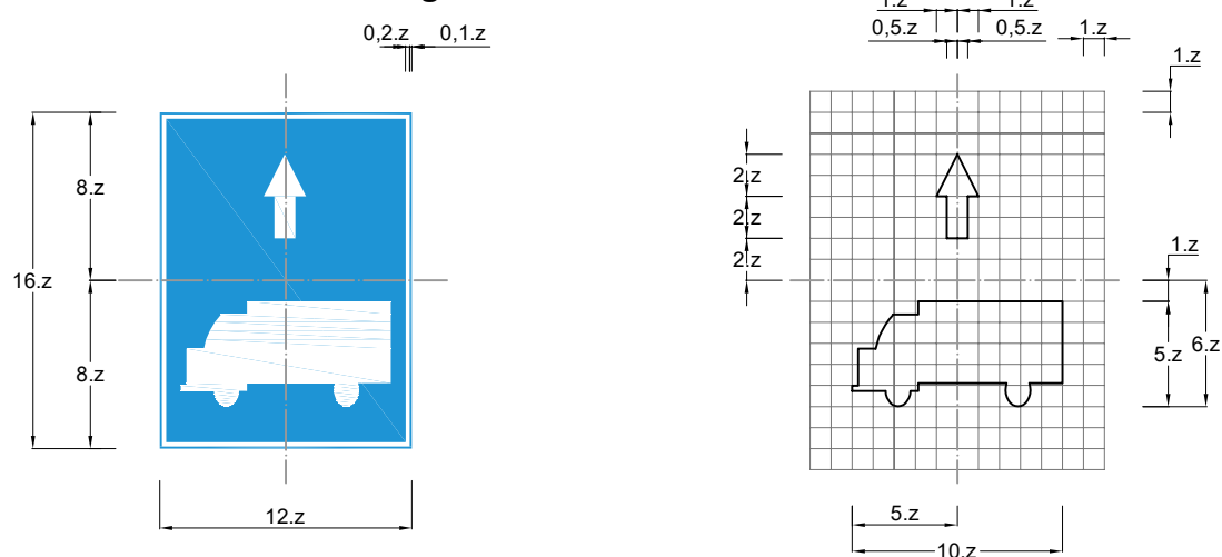
Biển số R.412c: Làn đường dành cho xe ô tô tải
