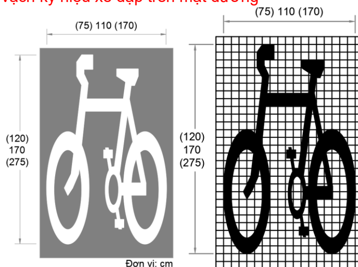
Hình G.82 - Vạch ký hiệu làn đường dành riêng cho xe đạp
