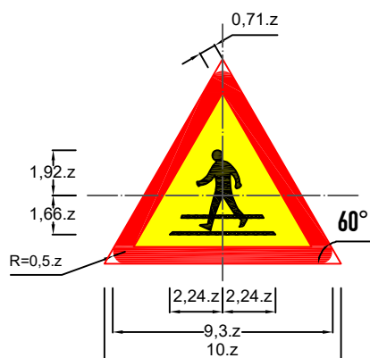
Biển số W.224: Đường người đi bộ cắt ngang
