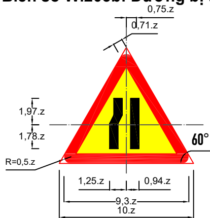
Biển số W.203b: Đường bị thu hẹp về phía trái
