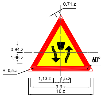
Biển số W.235: Đường đôi
