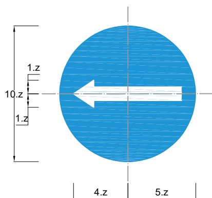
Biển số R.301c: Các xe chỉ được rẽ trái
