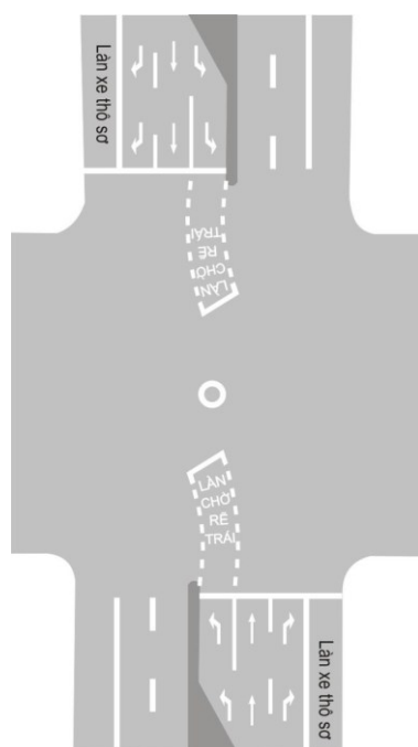
Hình G.42 - Minh họa bố trí vạch 5.3
