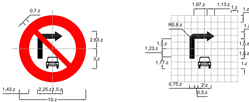
Biển số P.103b: Cấm xe ô tô rẽ phải
