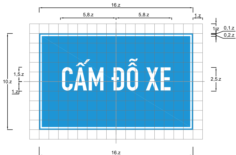
Biển số S.509b : Thuyết minh biển chính
