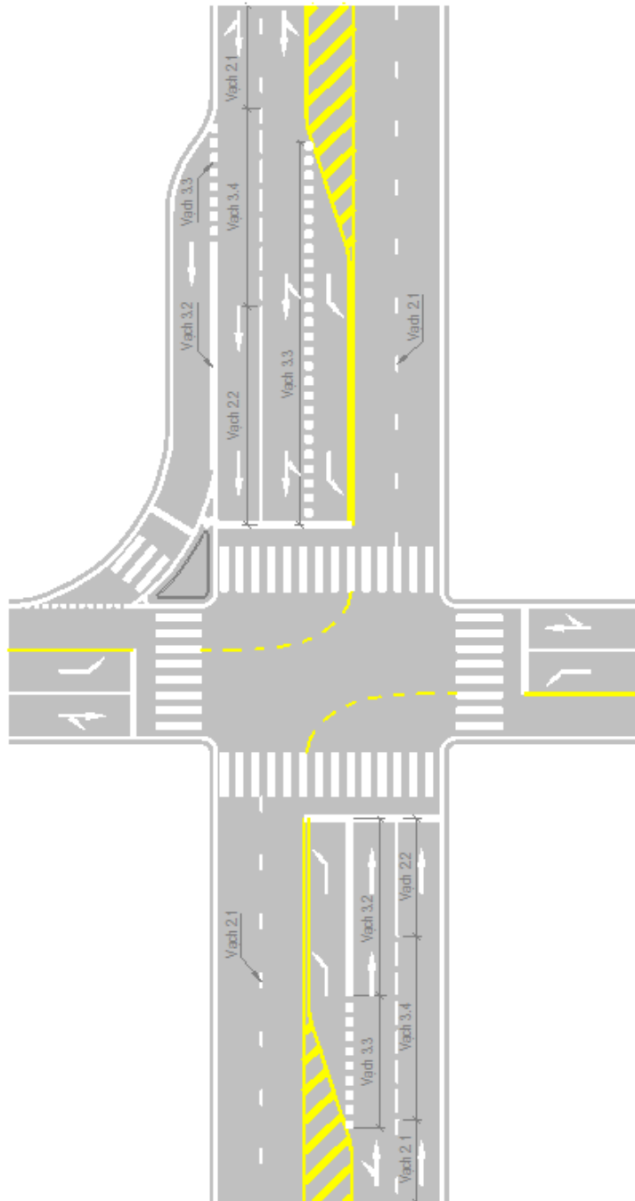
Hình G.43 - Minh họa bố trí phân làn đường trong khu vực nút giao cùng mức G1.6. Nhóm vạch cấm dừng xe trên đường a. Vạch 6.1: Vạch cấm đỗ xe trên đường
