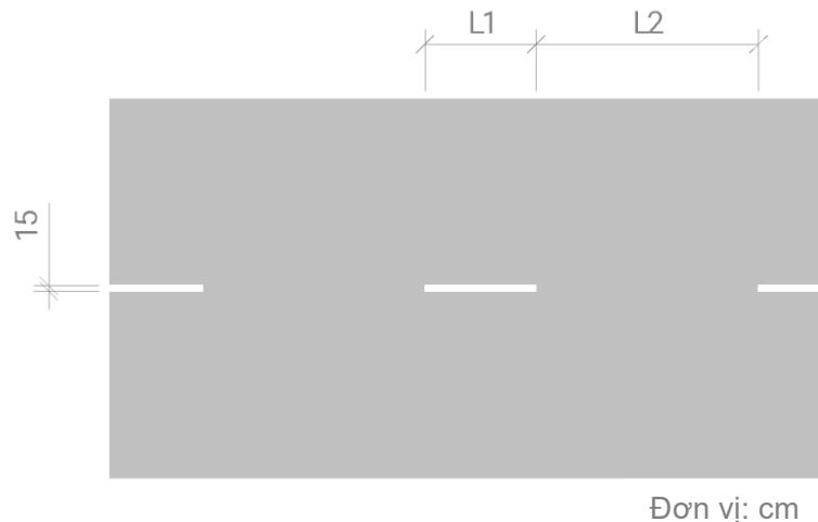
Hình G.10 - Vạch 2.1
