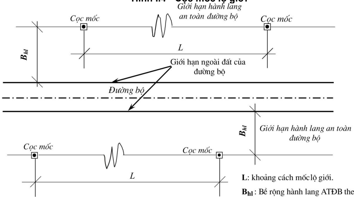
Hình I.4 - Cọc mốc lộ giới
