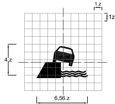
Biển số W.215b: Kè, vực sâu bên đường phía bên trái
