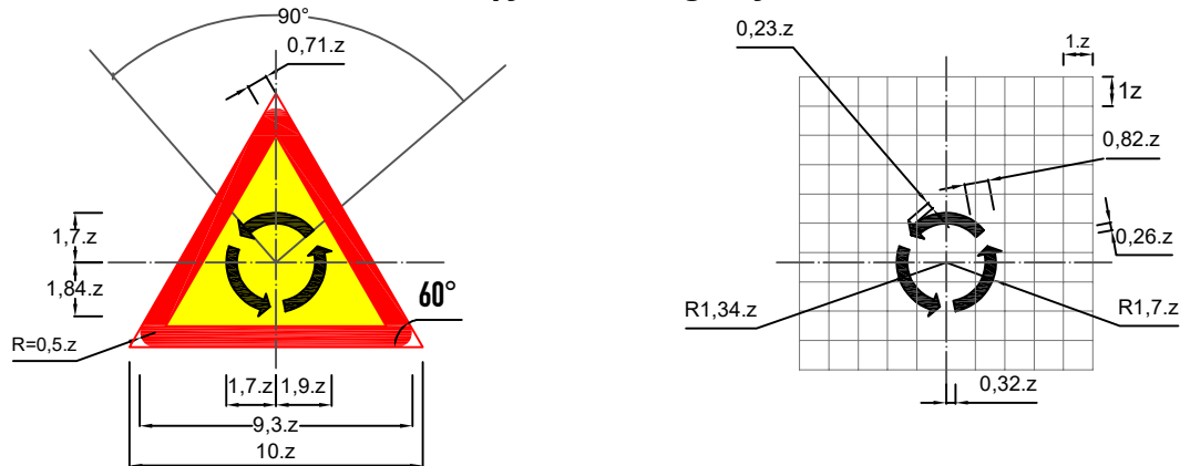
Biển số W.206: Giao nhau chạy theo vòng xuyến
