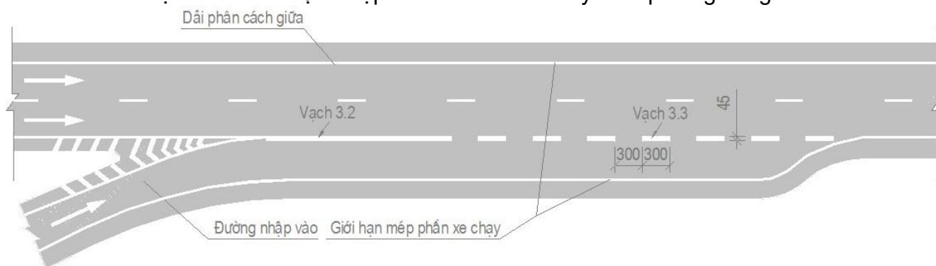
Hình G.16 - Minh họa bố trí vạch sơn khu vực nhập làn kiểu trực tiếp - Bố trí vạch sơn khu vực nhập làn kiểu có làn chuyển tiếp song song:
