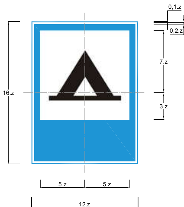
Biển số I.433b : Báo hiệu nơi cắm trại, nhà nghỉ lưu động
