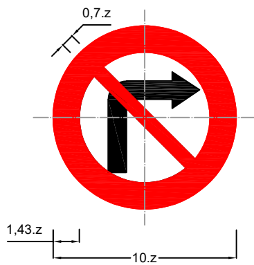
Biển số P.123b: Cấm rẽ phải
