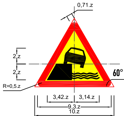
Biển số W.215b: Kè, vực sâu bên đường phía bên trái
