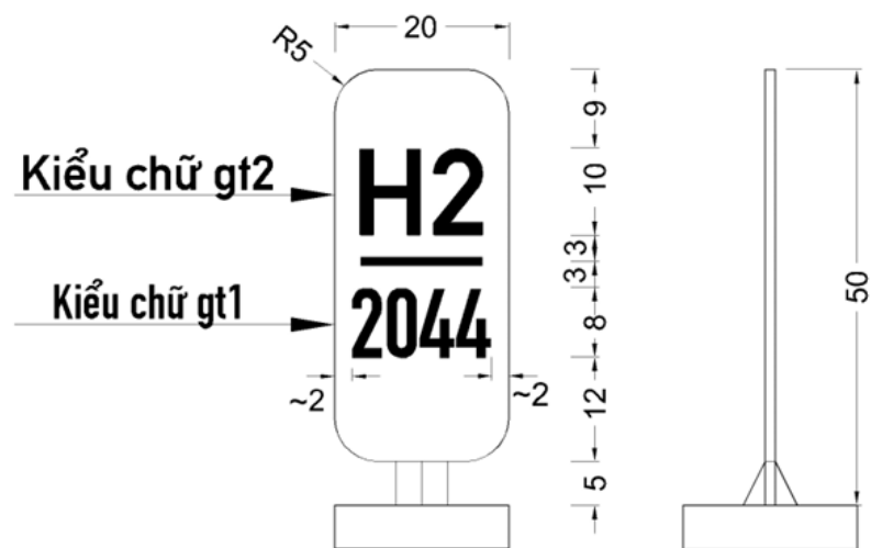
c) Cọc H dạng tấm, loại có ba và bốn chữ số lý trình Hình I.6 - Chi tiết cọc H
