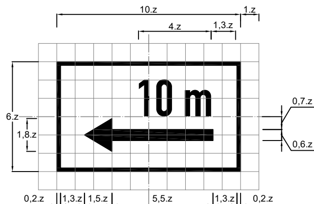
Biển SH.3a: Hướng tác dụng của biển
