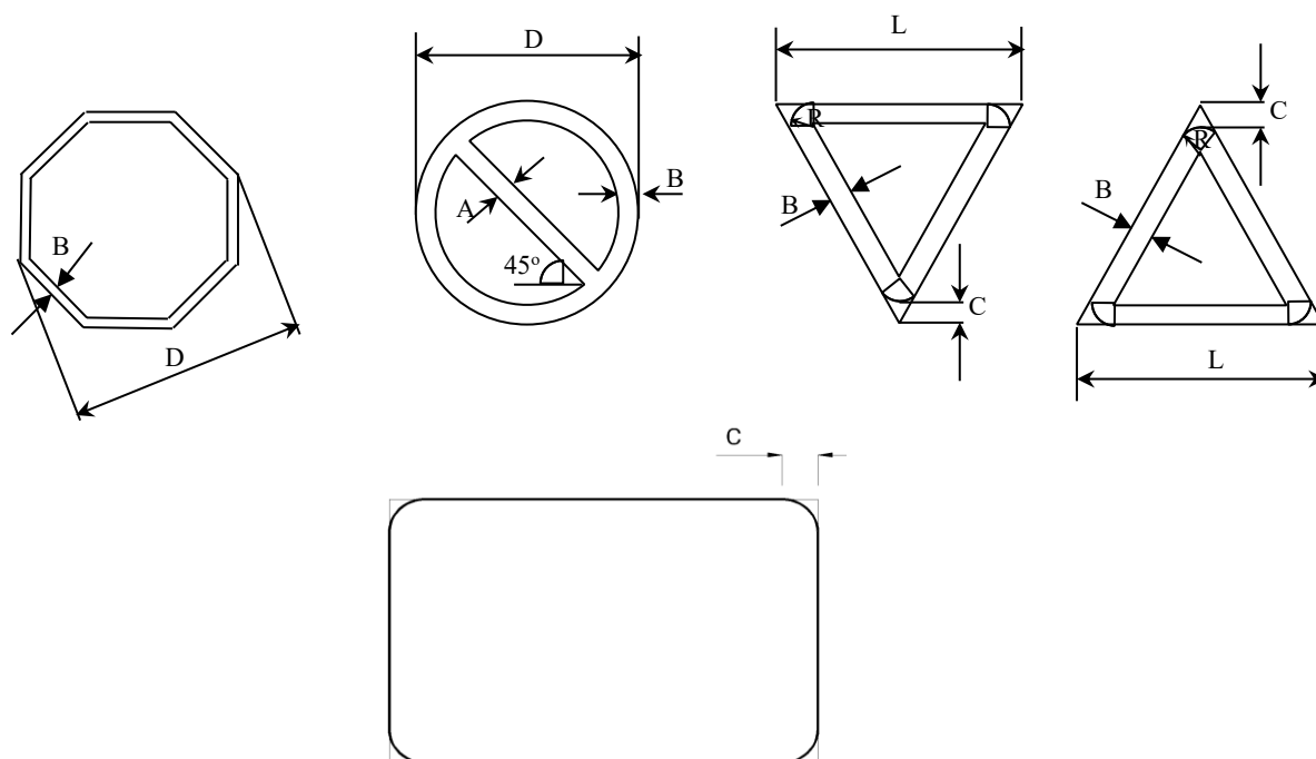
Hình 1 - Kích thước các loại biển báo
