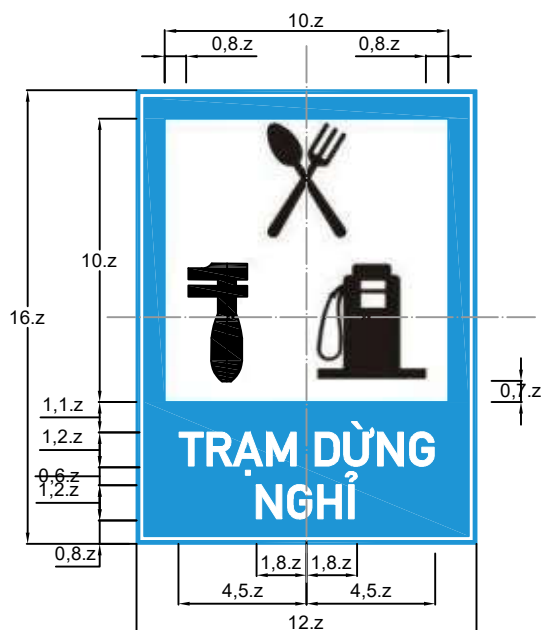
Biển số I.431 : Trạm dừng nghỉ
