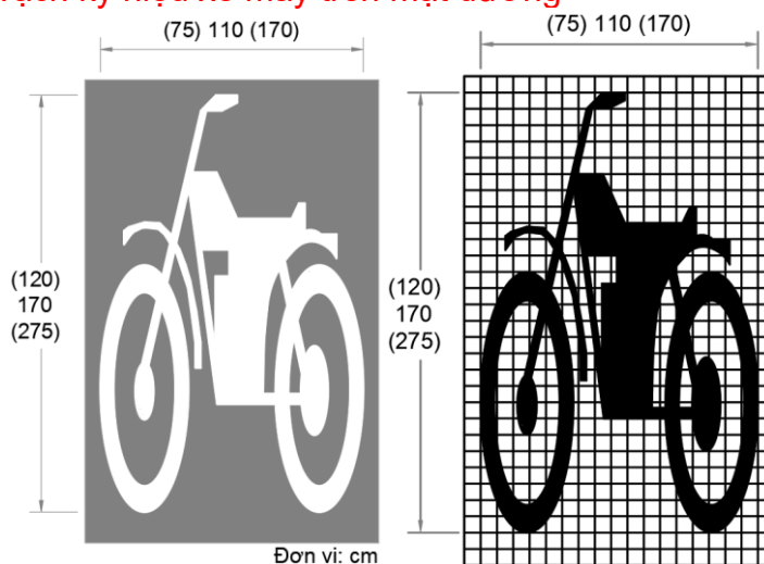
Hình G.83 - Vạch ký hiệu làn đường dành riêng cho xe máy
