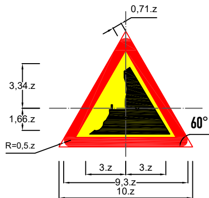
Biển số W.223b: Vách núi nguy hiểm
