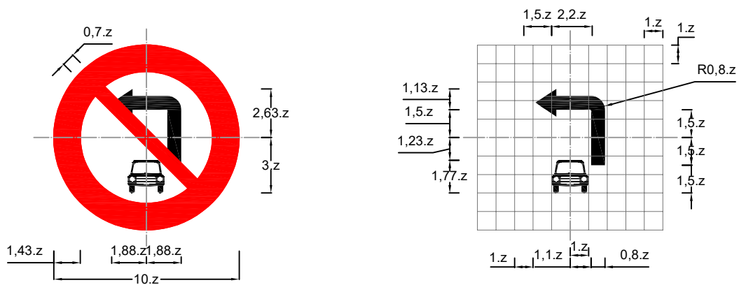
Biển số P.103c: Cấm xe ô tô rẽ trái
