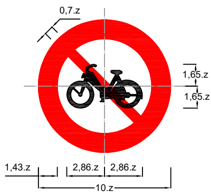
Biển số P.111a: Cấm xe gắn máy
