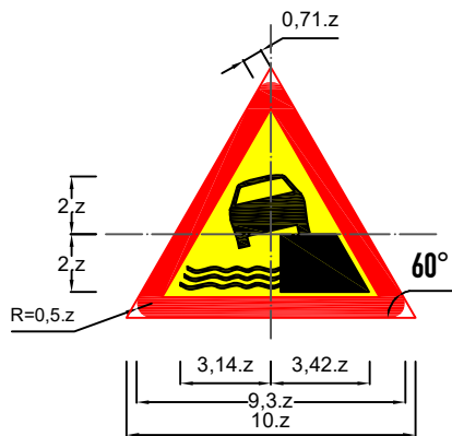
Biển số W.215c: Kè, vực sâu bên đường phía bên phải
