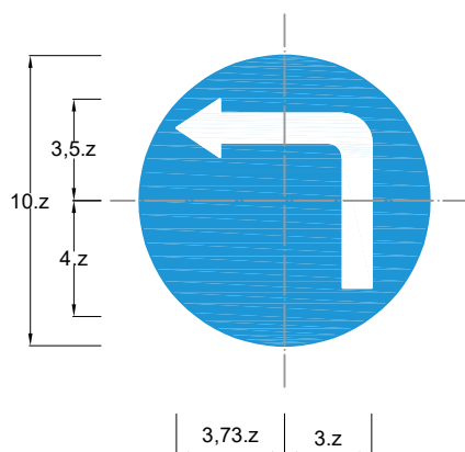
Biển số R.301e: Các xe chỉ được rẽ trái
