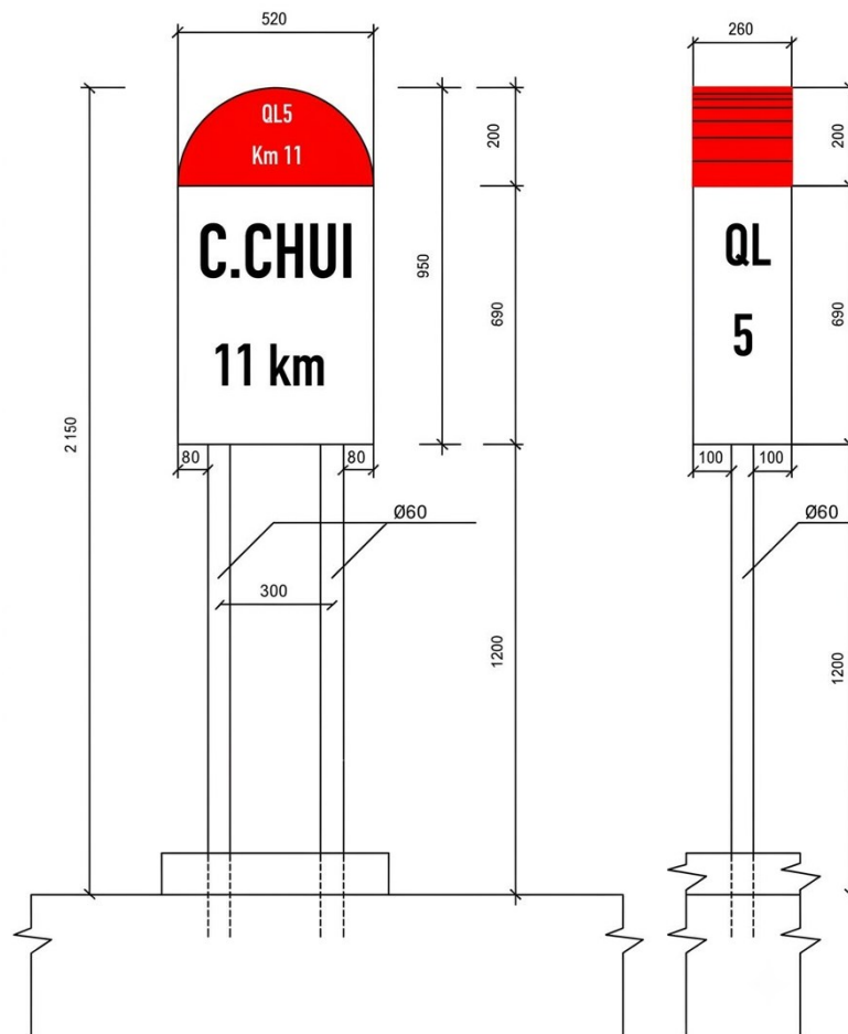
Hình I.2 - Cột kilômét dạng cột cao
