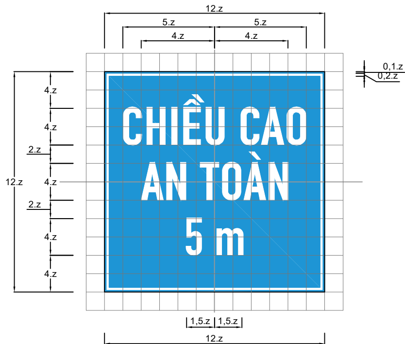
Biển số S.509b : Thuyết minh biển chính
