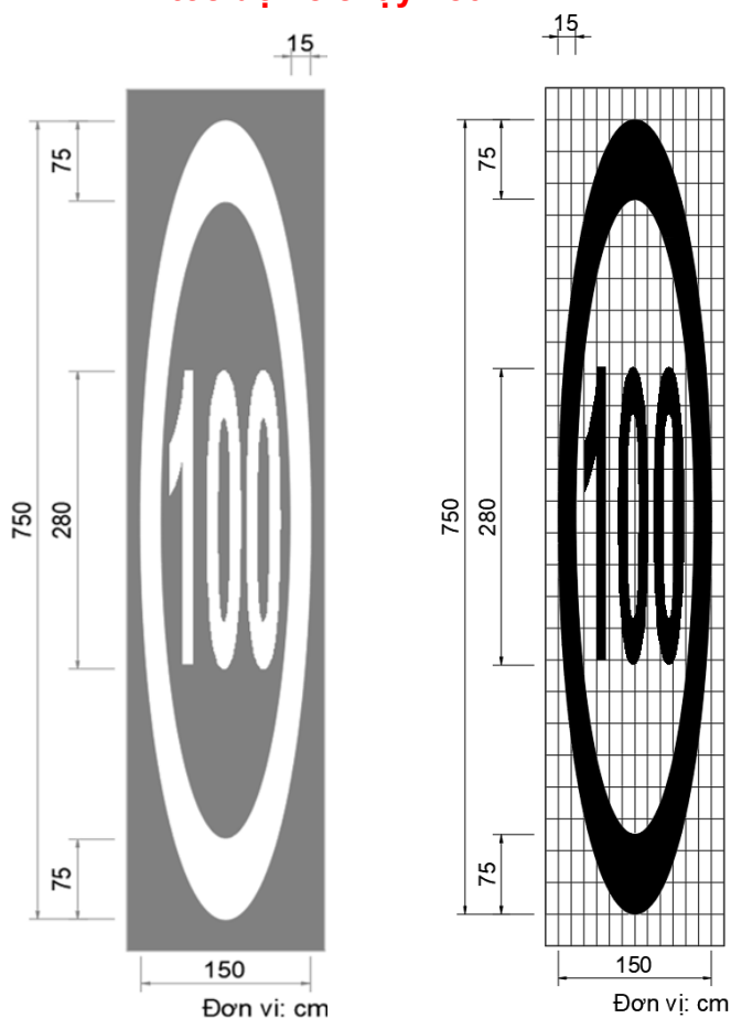
Hình G.86 - Vạch sơn tốc độ tối đa cho phép trên mặt đường áp dụng cho đường có tốc độ xe chạy \geq 80 km/h
