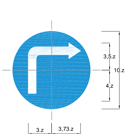
Biển số R.301d: các xe chỉ được rẽ phải
