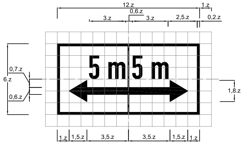
Biển SH.3b : Hướng tác dụng của biển
